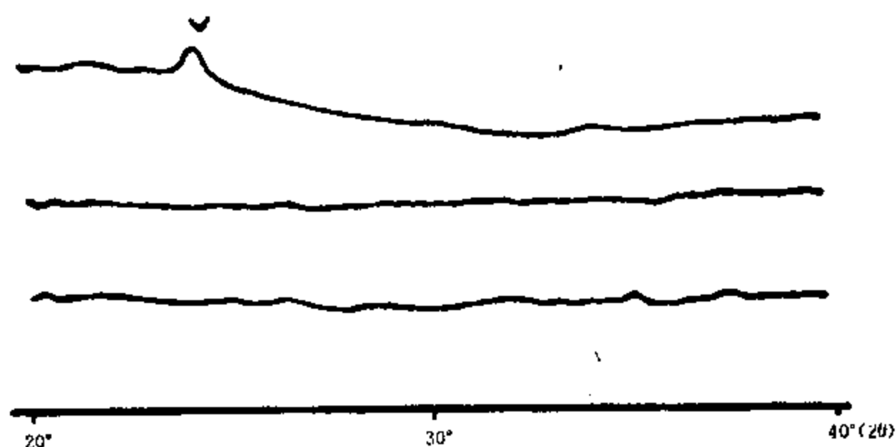
图 15 下-4-3 联苯双酯-PVP 物理混合物及固体分散物 X-射线衍射图 箭头指示联苯双酯晶体衍射峰
