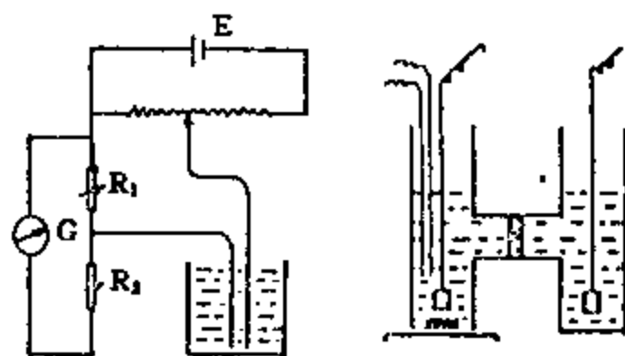
图 12-3-4 仪器装置
