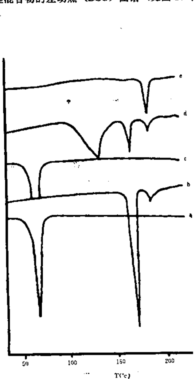
图 15 下-4-5 三种联苯双酯制剂的 DTA 图 a. PEG6000; b. 联苯双酯; c. 联苯双酯滴丸; d. 联苯双酯片 I; e. 联苯双酯片 II
