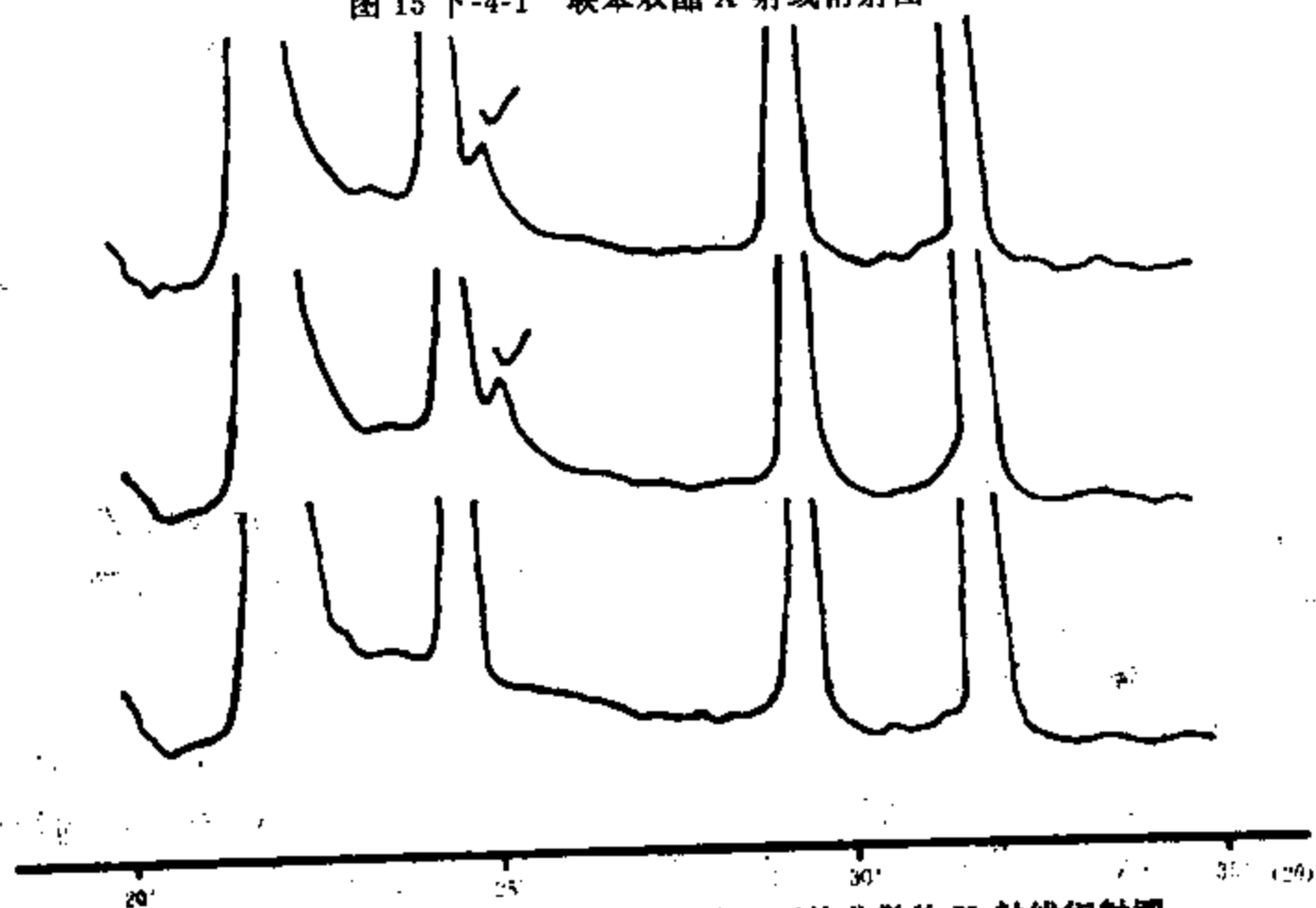
图 15 下-4-2 联苯双酯-PEG物理混合物及固体分散物 X-射线衍射图
