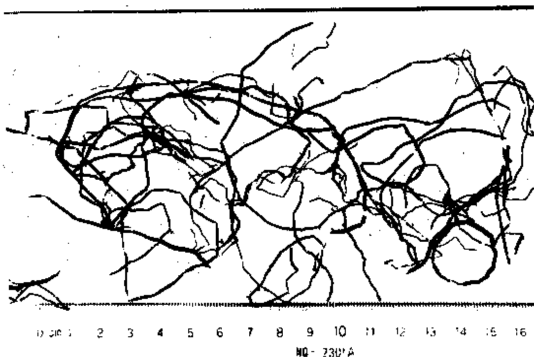
图 2-1-4 自然条件下蜜环菌菌索
