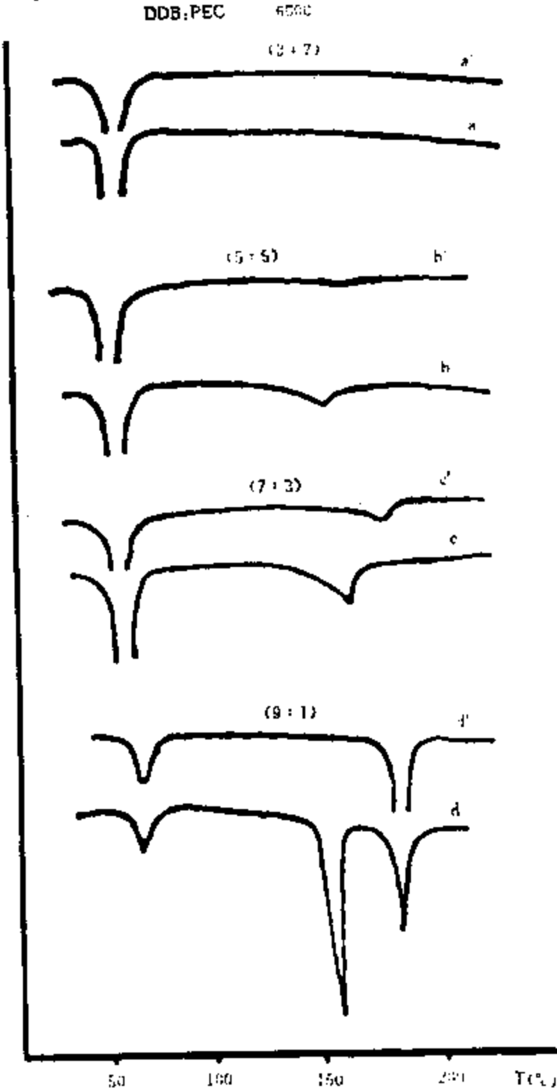
图 15 下-4-6 联苯双酯-PEG6000 物理混合物及 固体分散物的 DSC 图 a, b, c, d: 物理混合物; a', b', c', d': 固体分散物
