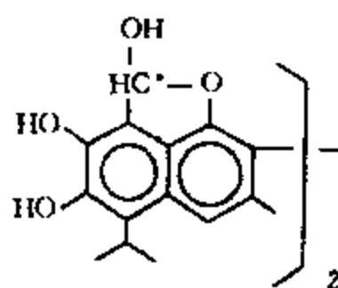
图 8-2-6 棉酚内醚结构
