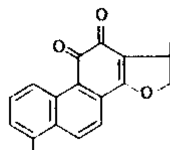
二氢丹参酮 I
