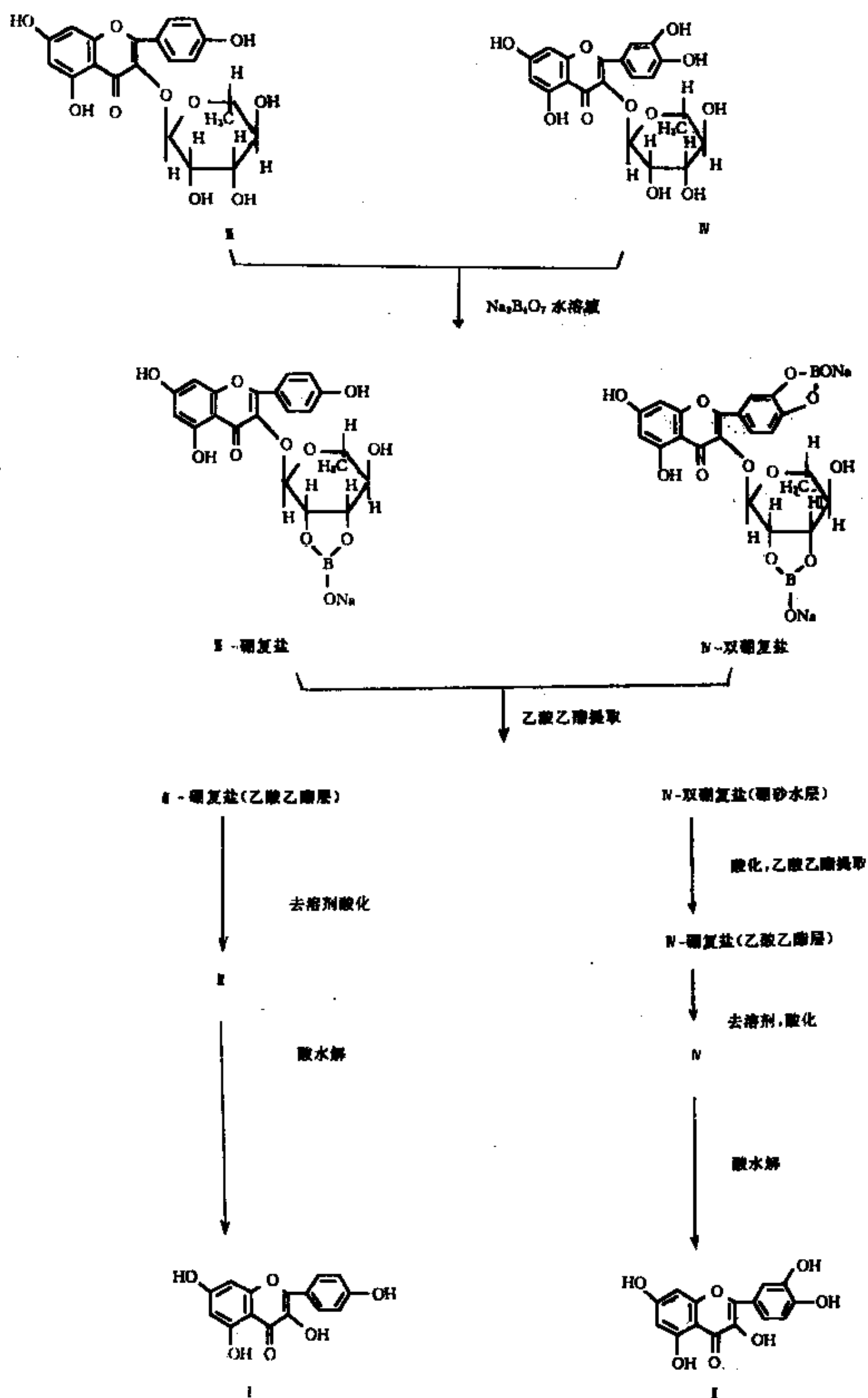
图 5-2-1 猫眼草总黄酮分离路线
