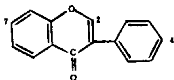
图 12-2-3 大豆甙元的基本骨架
