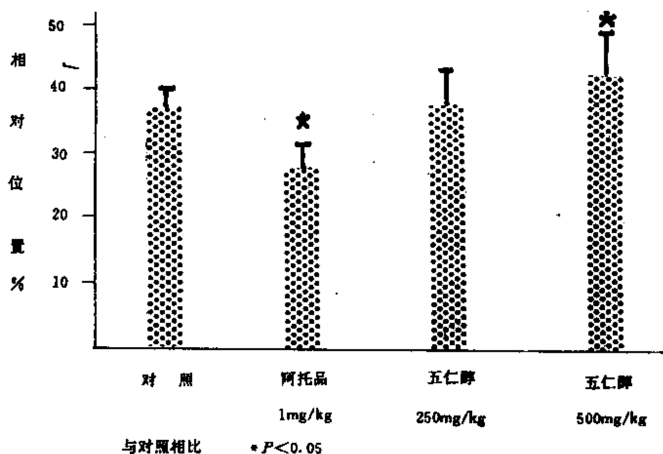
图 15 上-3-1 五仁醇对小鼠胃肠运动的影响
