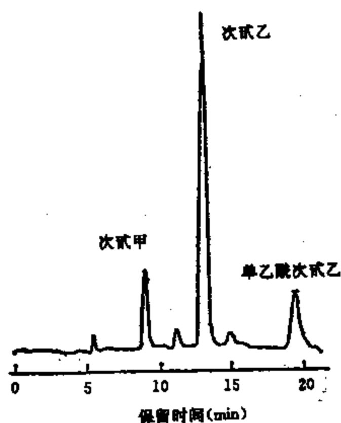
图 16-3-7 黄夹甙 HPLC 图谱
