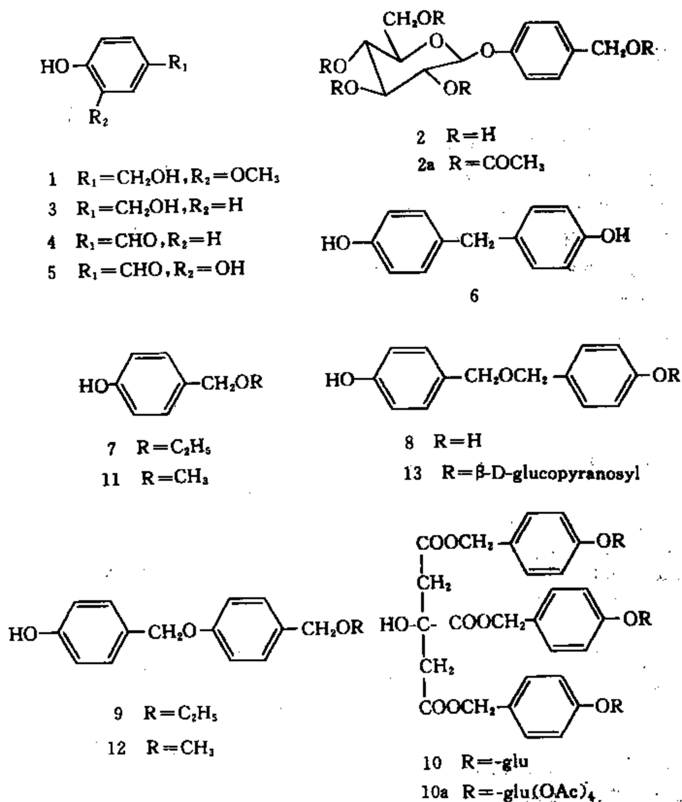
图 6-3-1 天麻中提取分离化合物的结构图
