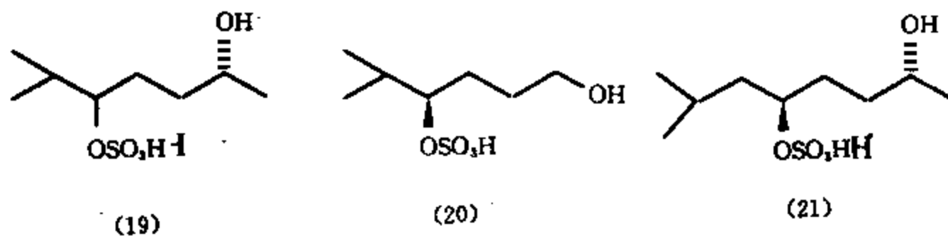
图 10-2-4 麝香中具强心作用成分
