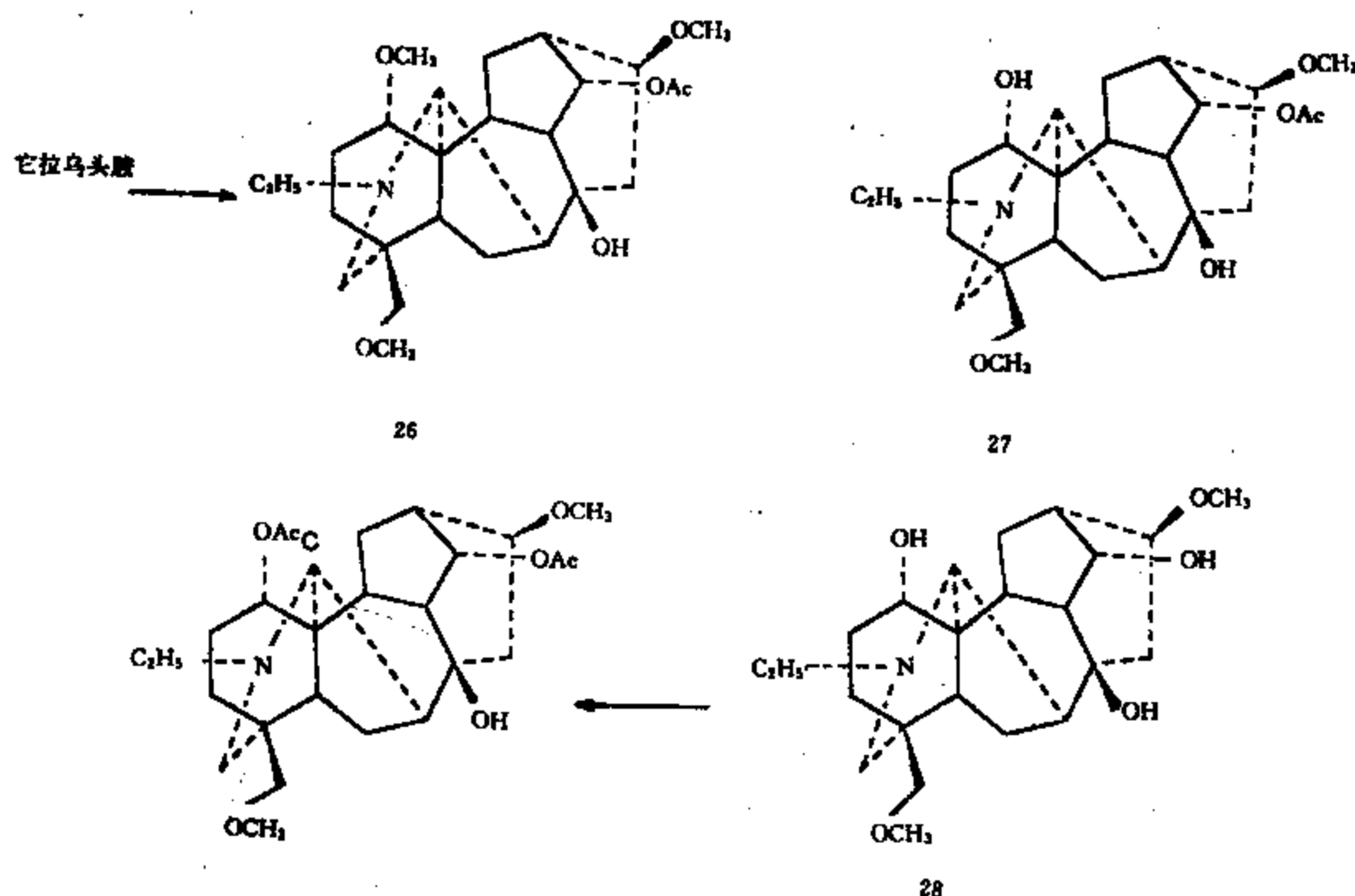
图 1-2-11 它拉乌头胺 (16) 乙酰它拉乌头胺 (26) 乱飞燕草碱 (27) 和异它拉乌头定 (28) 之间的结构关系
