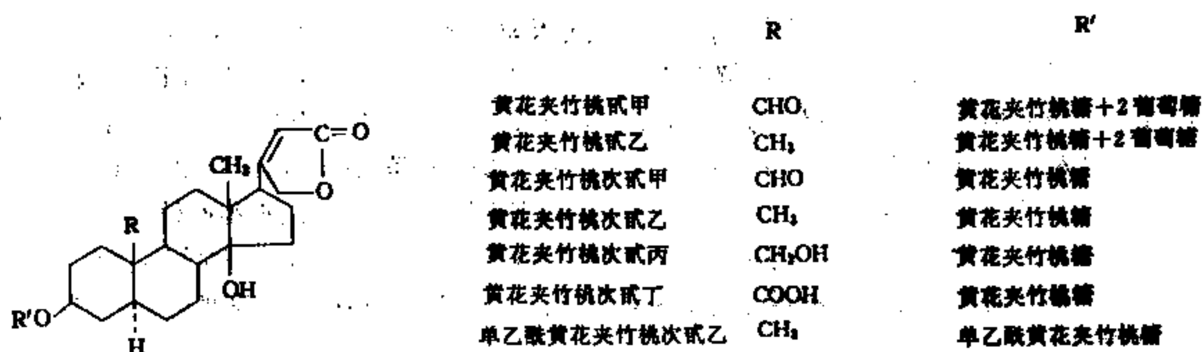
图 5 黄花夹竹桃中七种强心甙结构
