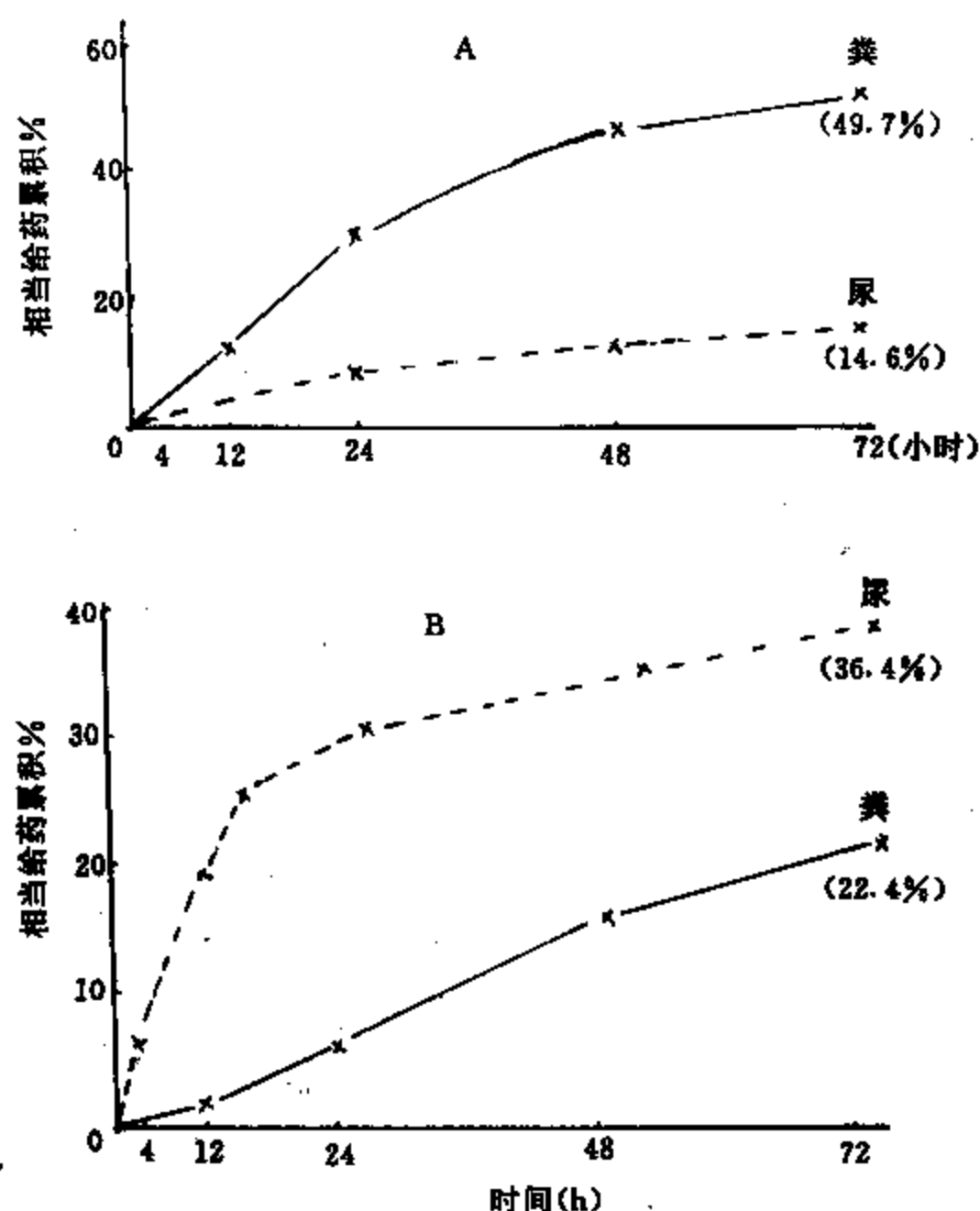
图 11-4-3 ^3\text{H} -甲异靛与 ^3\text{H} -靛玉红口服给药后排泄的比较 A. 靛玉红; B. 甲异靛
