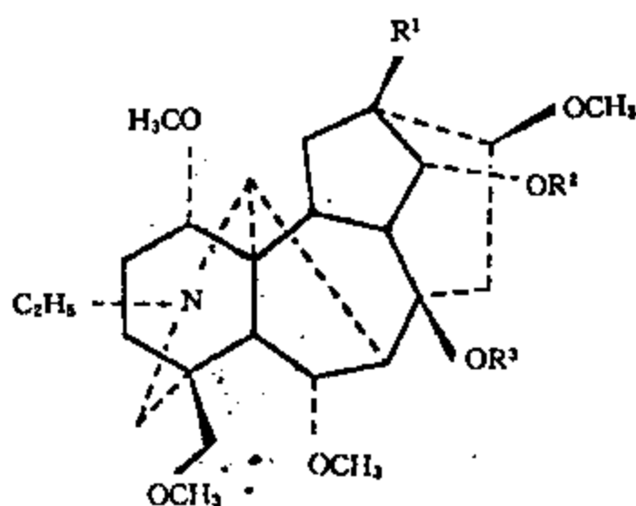
图1-2-4 丽乌碱 (7) 的化学结构
