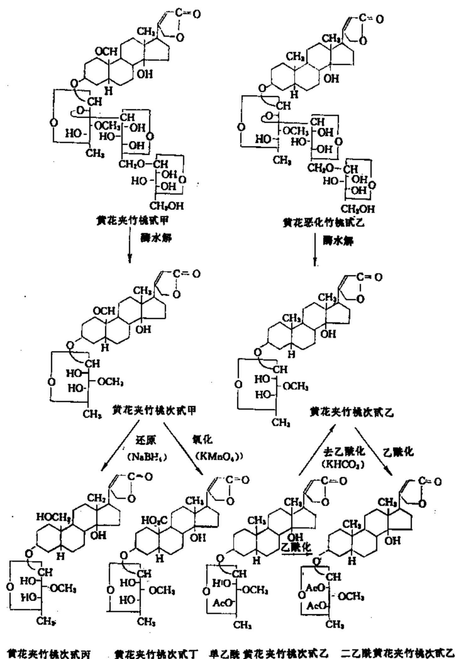
图 16-2-1 黄花夹竹桃中强心甙的结构
