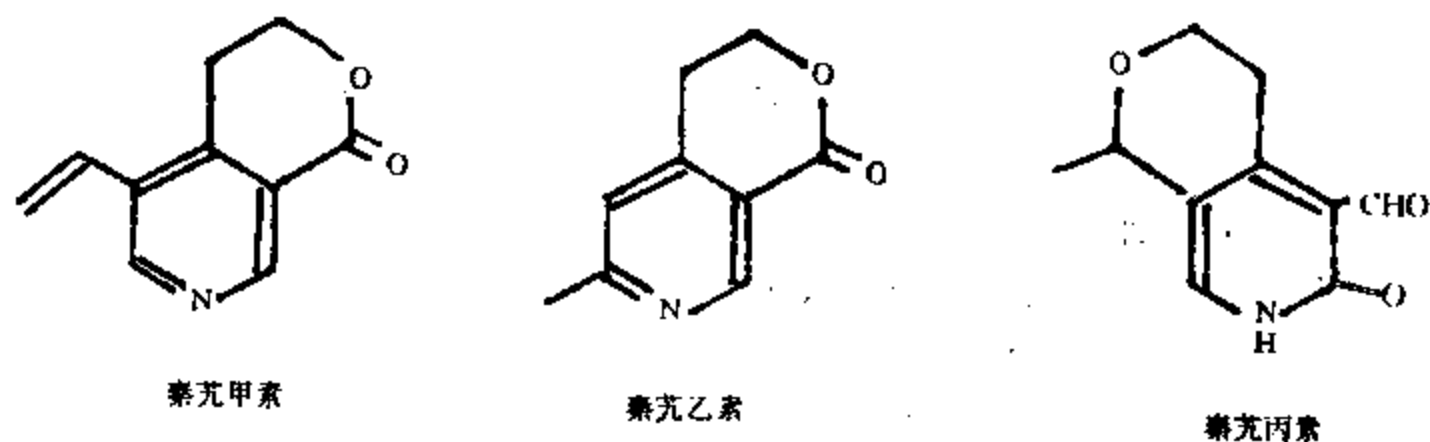
图 7-2-1 秦艽中的生物碱
