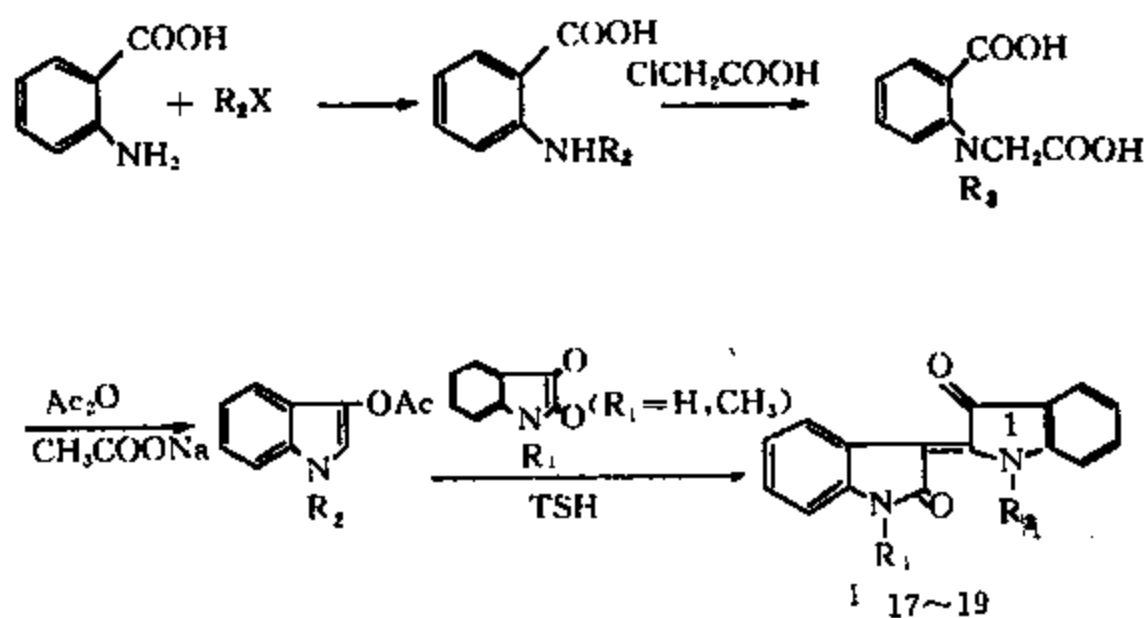
图 11-2-6 赭玉红衍生物 I 17~19 的合成路线
