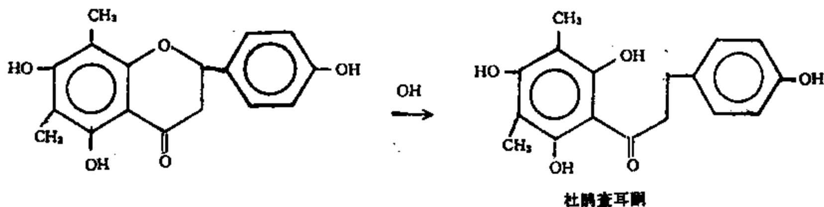
图 14-4-2 杜鹃素与碱反应式
