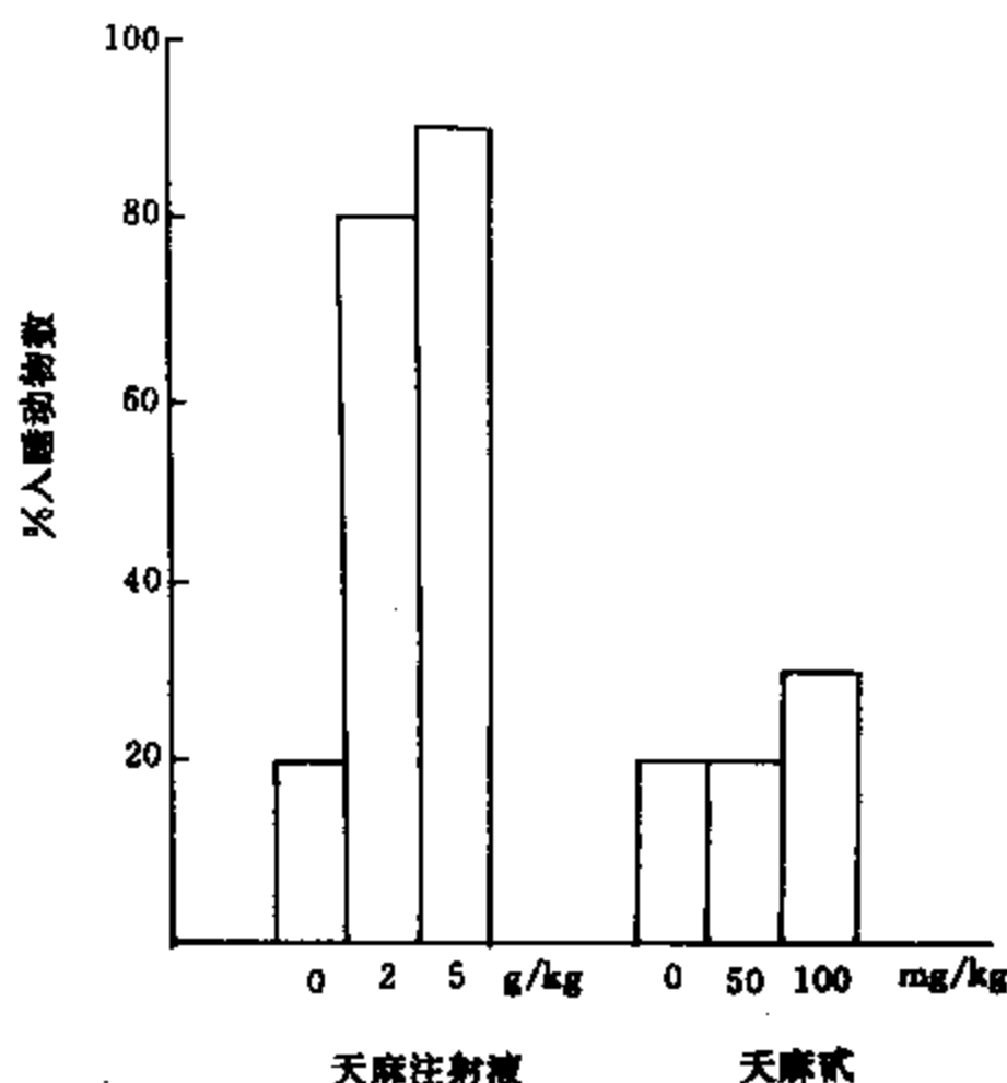
图 6-4-1 对阈下剂量戊巴比妥钠作用的影响
