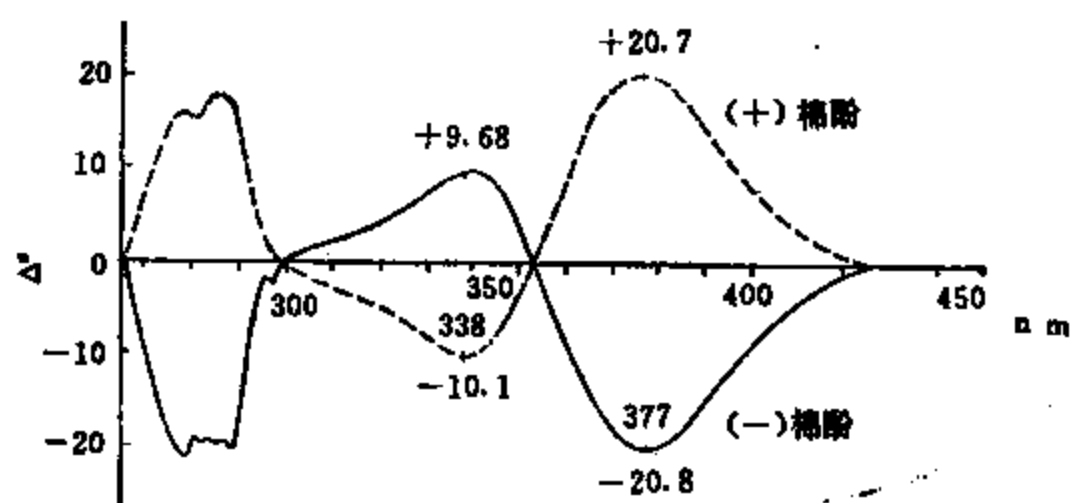
图 8-2-8 (+)、(-) 棉酚的 CD 光谱
