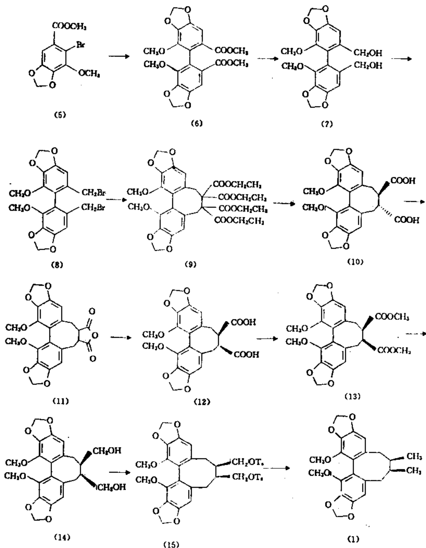
图 15 下-1-2 五味子丙素人工全合成路线
