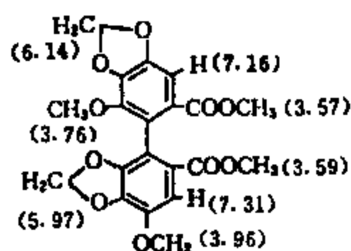
\beta -联苯双酯 (27)
