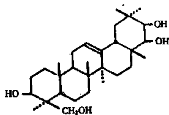
25 大豆皂甙元 A
