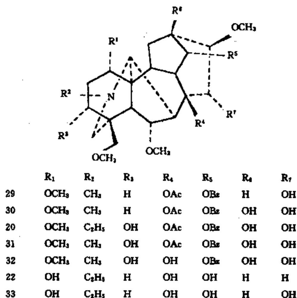
图 1-2-12 异翠雀碱 (29) 次乌头碱 (30) 中乌头碱 (31) 苯甲酰中乌头原碱 (32) 羟基新乌碱 (33) 的结构
