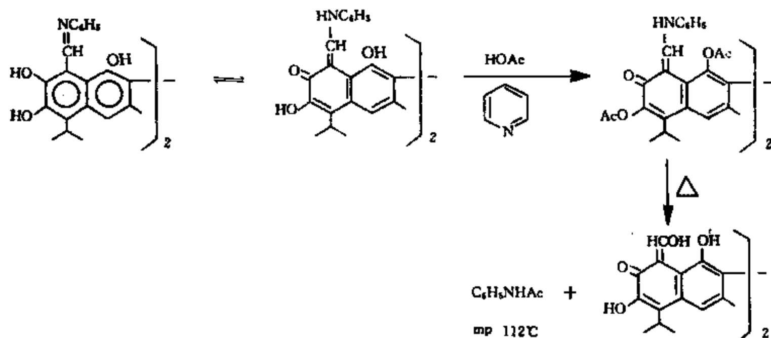
图 8-2-4 双苯胺棉酚受热失去乙酰苯胺
