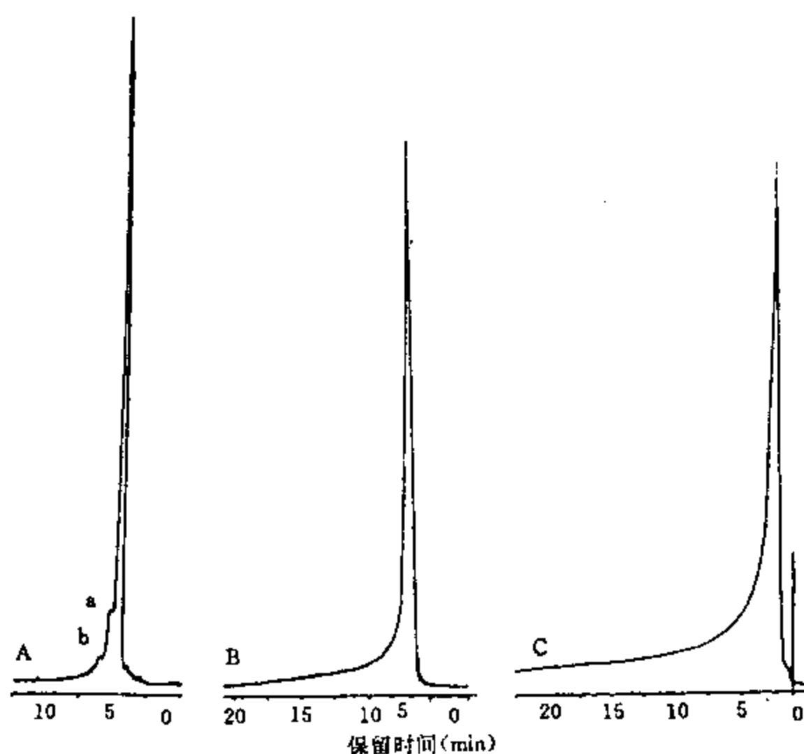
图 8-3-1 醋酸棉酚用不同流动相层析的色谱图
