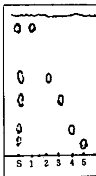
图 16-3-1 黄夹甙的纸色谱
