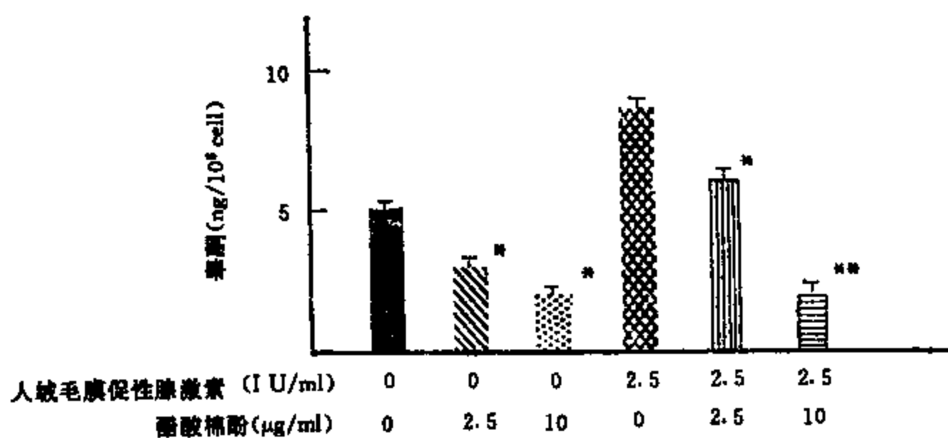
图 8-4-2 棉酚对大鼠间质细胞体外分泌睾酮的影响
