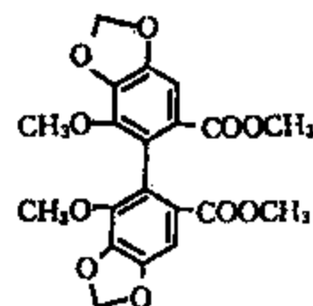
\gamma -联苯双酯 (28)
