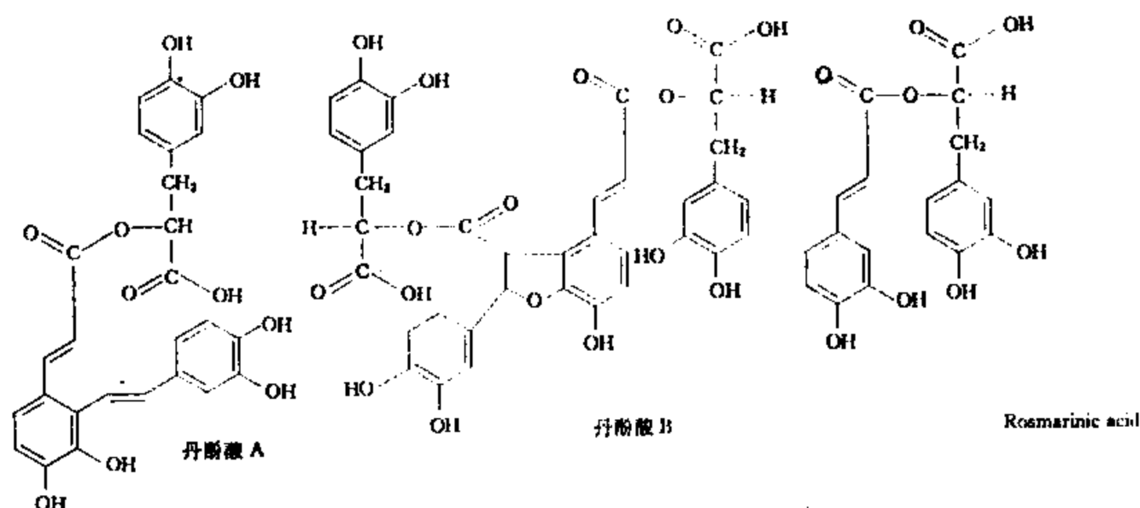
图 13 三种丹酚酸结构
