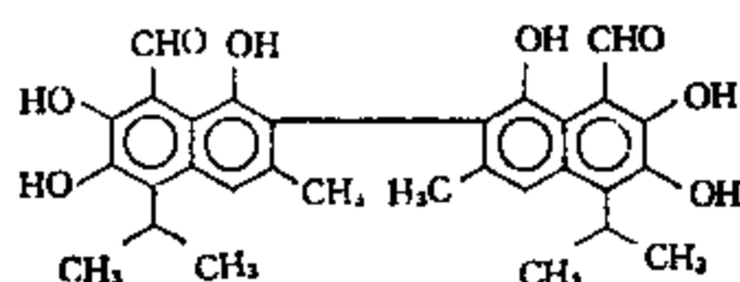
图 8-2-1 棉酚的结构式
