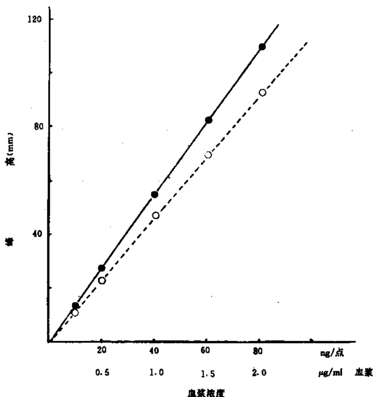
图 12-6-3 大豆甙元经高效薄层色谱—紫外扫描标准曲线
