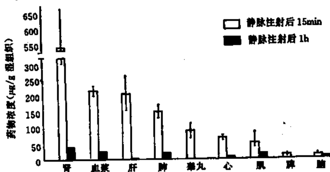
图 12-6-12 大鼠 iv 葛根素 15mg/kg 后药物的组织分布 (三只动物均值±SE, 血浆为 μg/ml)
