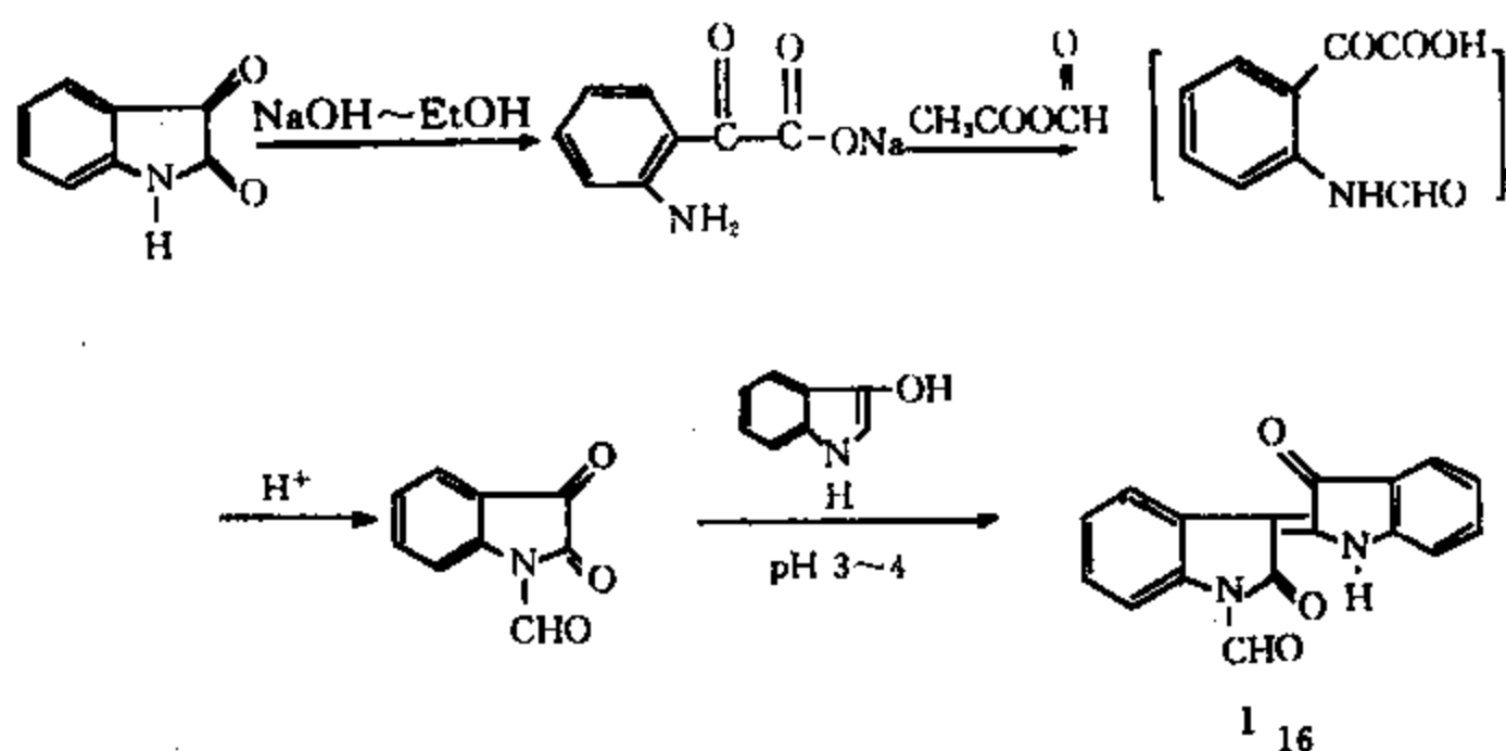
图 11-2-5 赭玉红衍生物 I 16 的合成路线
