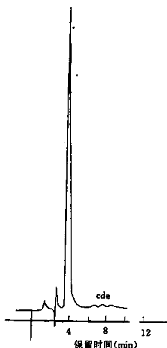
图 8-3-2 棉酚在 -\text{SO}_3\text{H} 柱上的色谱分离
