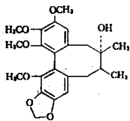
五味子醇乙
