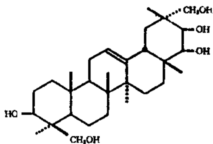
27 葛根甙元 A
