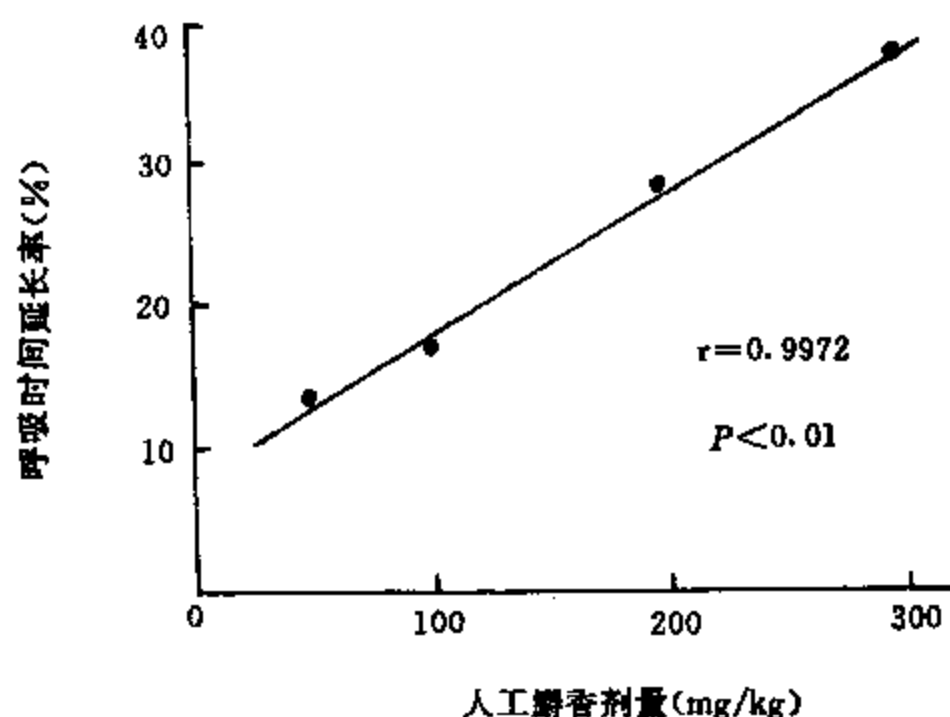
图 10-4-1 人工麝香对小鼠抗缺氧作用的量-效关系
