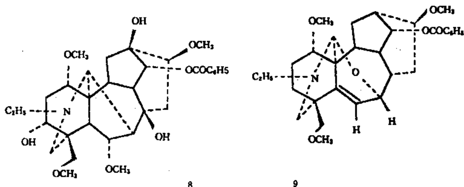
图 1-2-6 卢乌碱 (8) 及大渡乌碱 (9) 的结构
