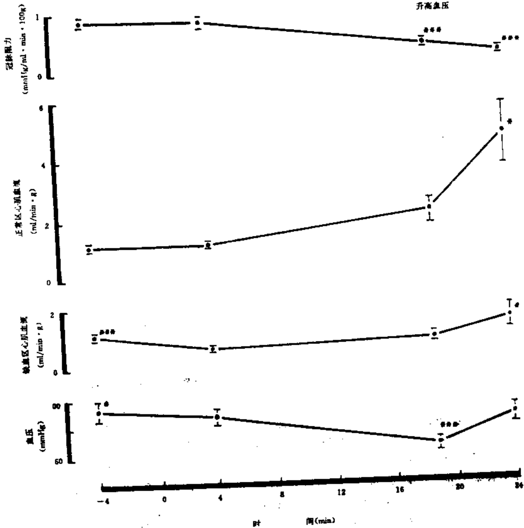
图 12-4-3 葛根素对急性心肌缺血狗区域性心肌血流的影响 (n=6) 与给药前 (即阻断冠脉 4min 后) 比较 *P<0.05 ***P<0.001
