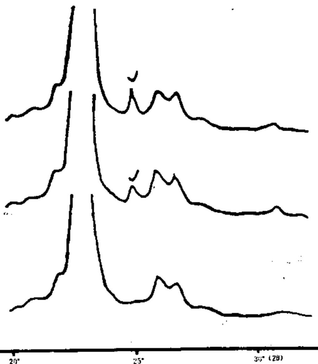
图 15 下-4-4 联苯双酯-PEG6000 物理混合物及固体分散物 X-射线衍射图 箭头指示联苯双酯晶体衍射峰
