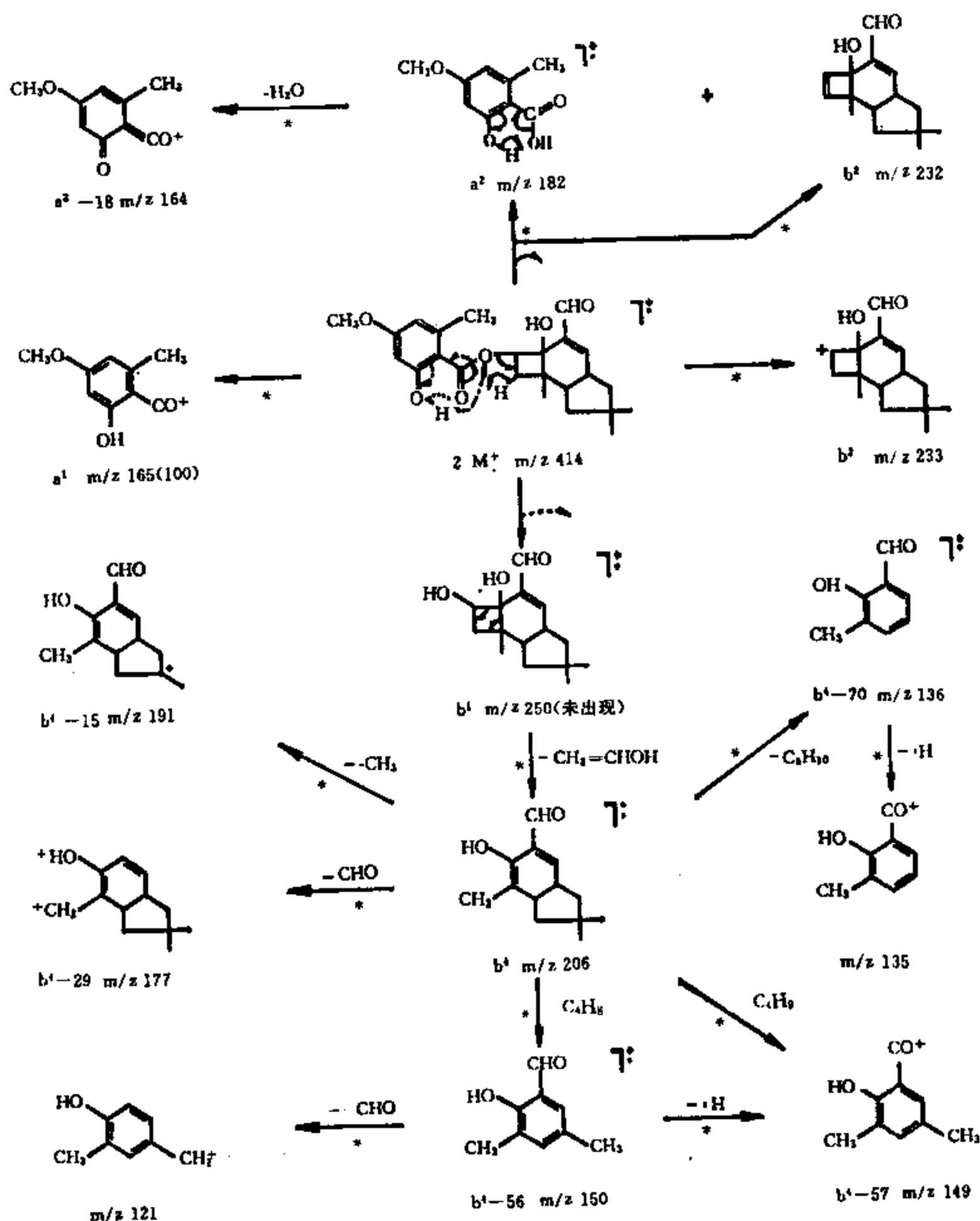
图 2-3-2 化合物 (1) 的质谱裂解方式 * 表示由亚稳离子证明 (下同)
