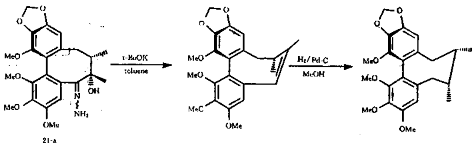
图 15 上-2-2 五味子乙素的半合成
