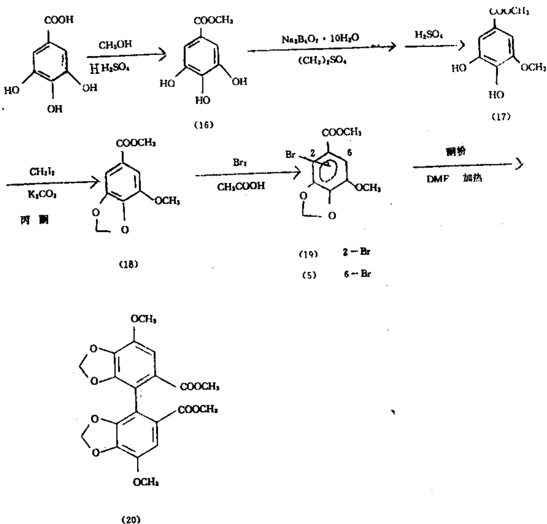
图15下-2-1 治疗慢性肝炎药联苯双酯的合成路线
