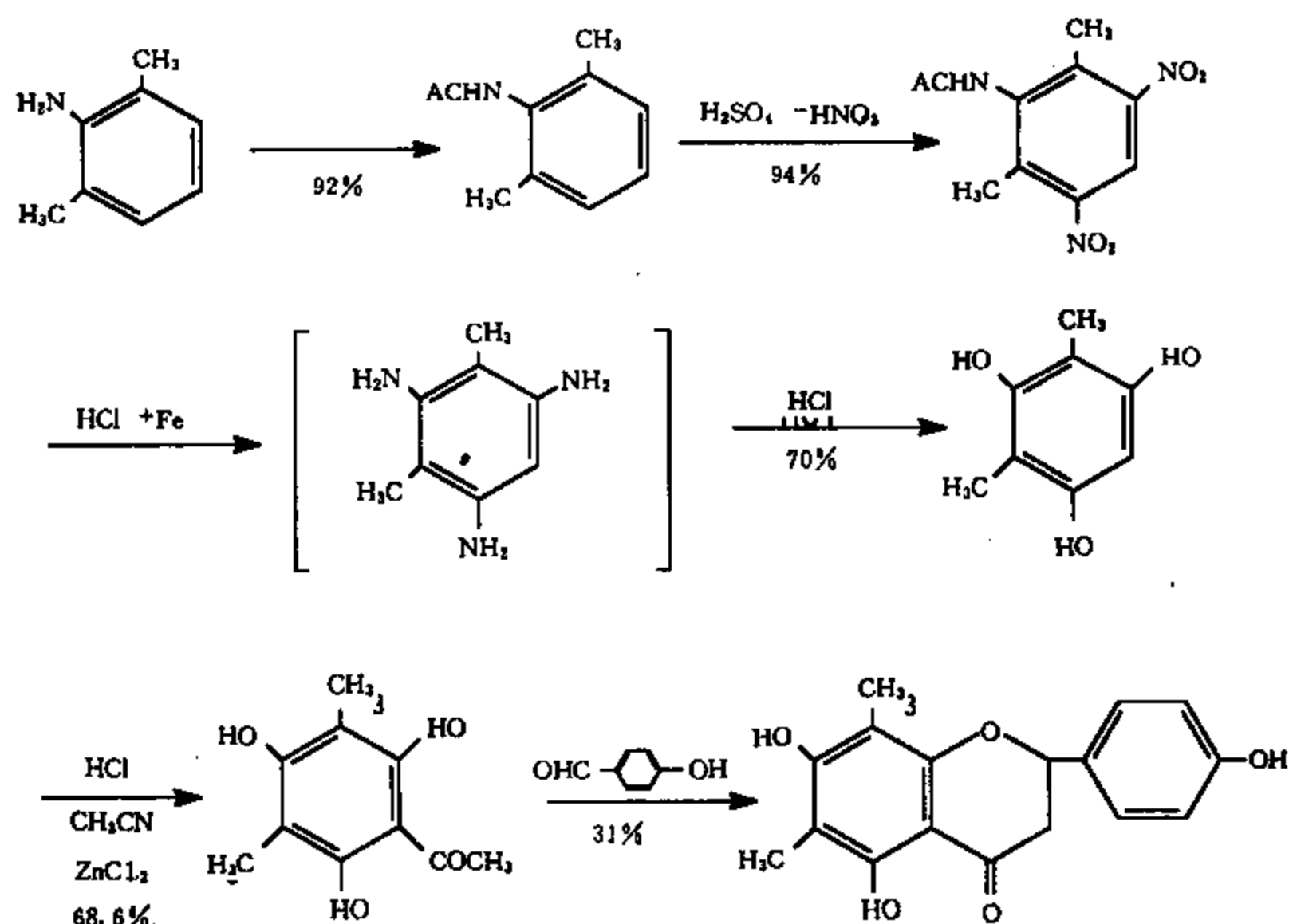
图 14-3-3 杜鹃素合成方法B
