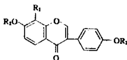
图 6 葛根黄酮结构
