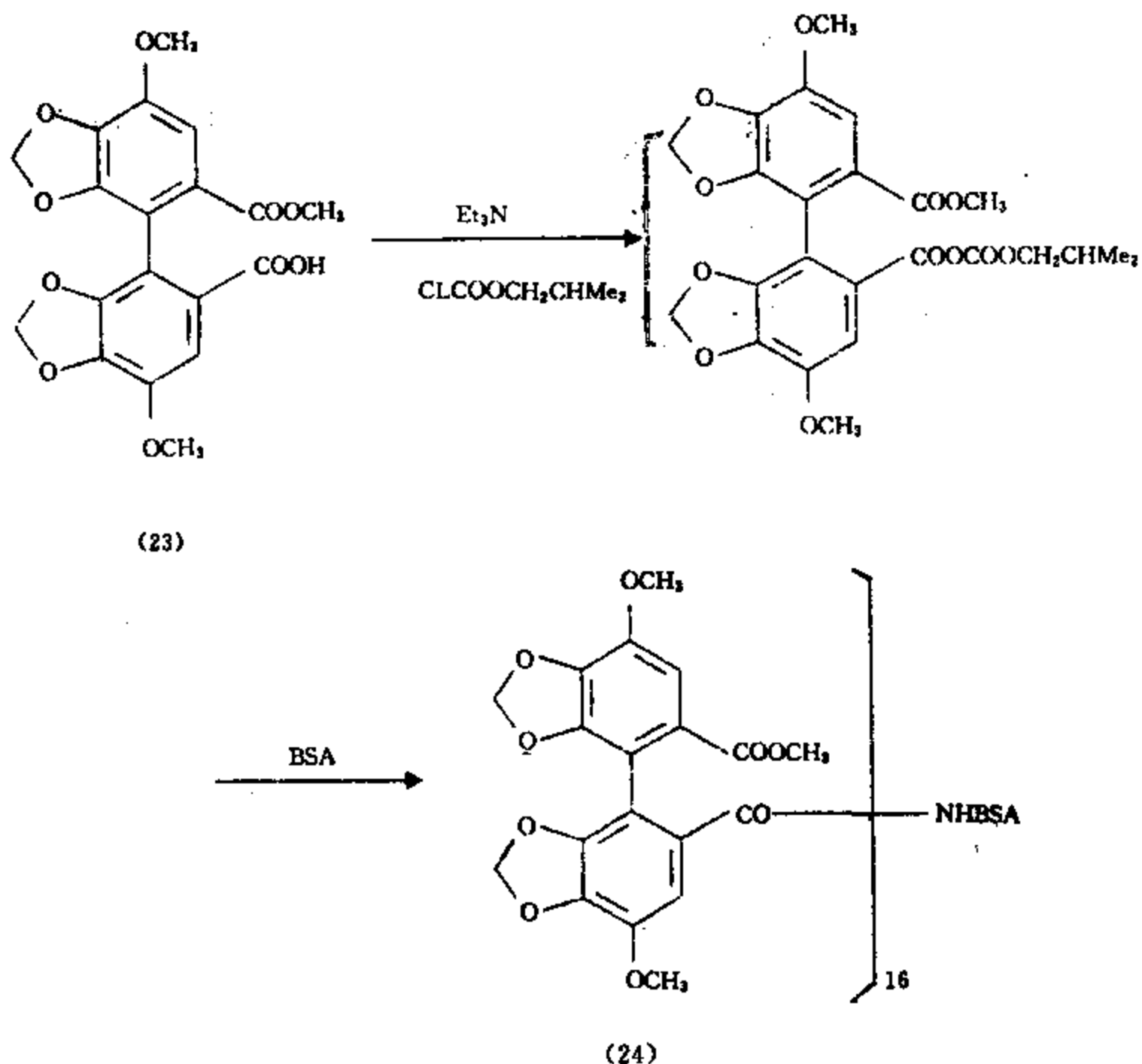
图 15 下-2-3 联苯双酯牛血清蛋白复合物的合成路线
