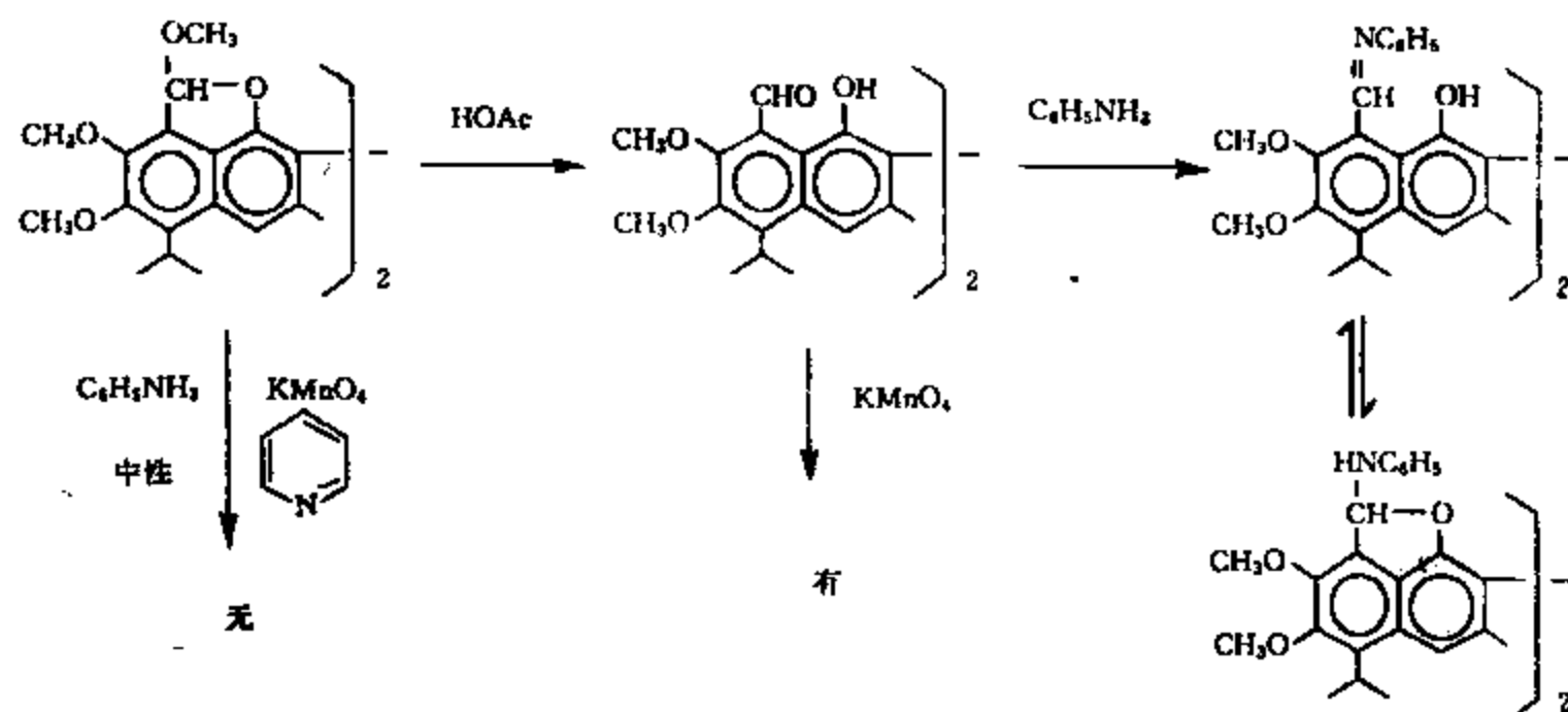
图 8-2-3 棉酚六甲醚的反应
