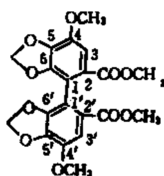
\alpha -联苯双酯 (20)
