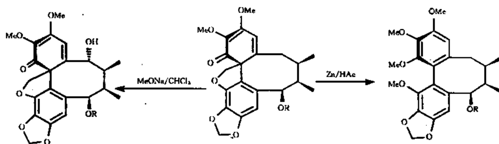
图 15 上-2-3 南五脂酮类木脂素的化学转变
