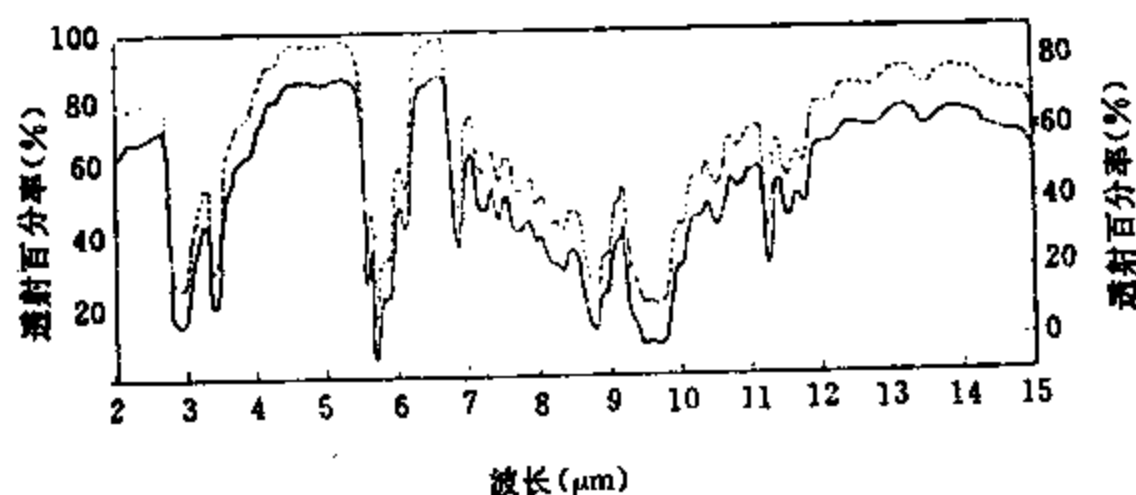
图 16-2-2 黄花夹竹桃次甙丁的红外吸收光谱 (KBr)
