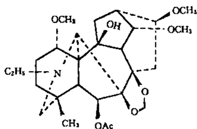
图 1-2-17 安莨菪牛扁碱 (67) 翠雀瓦因 (68) 去甲翠雀瓦因 (59、60) 混合物和翠雀它灵 (69) 核替辛 (70) 翠雀酰胺 (71) 的结构
