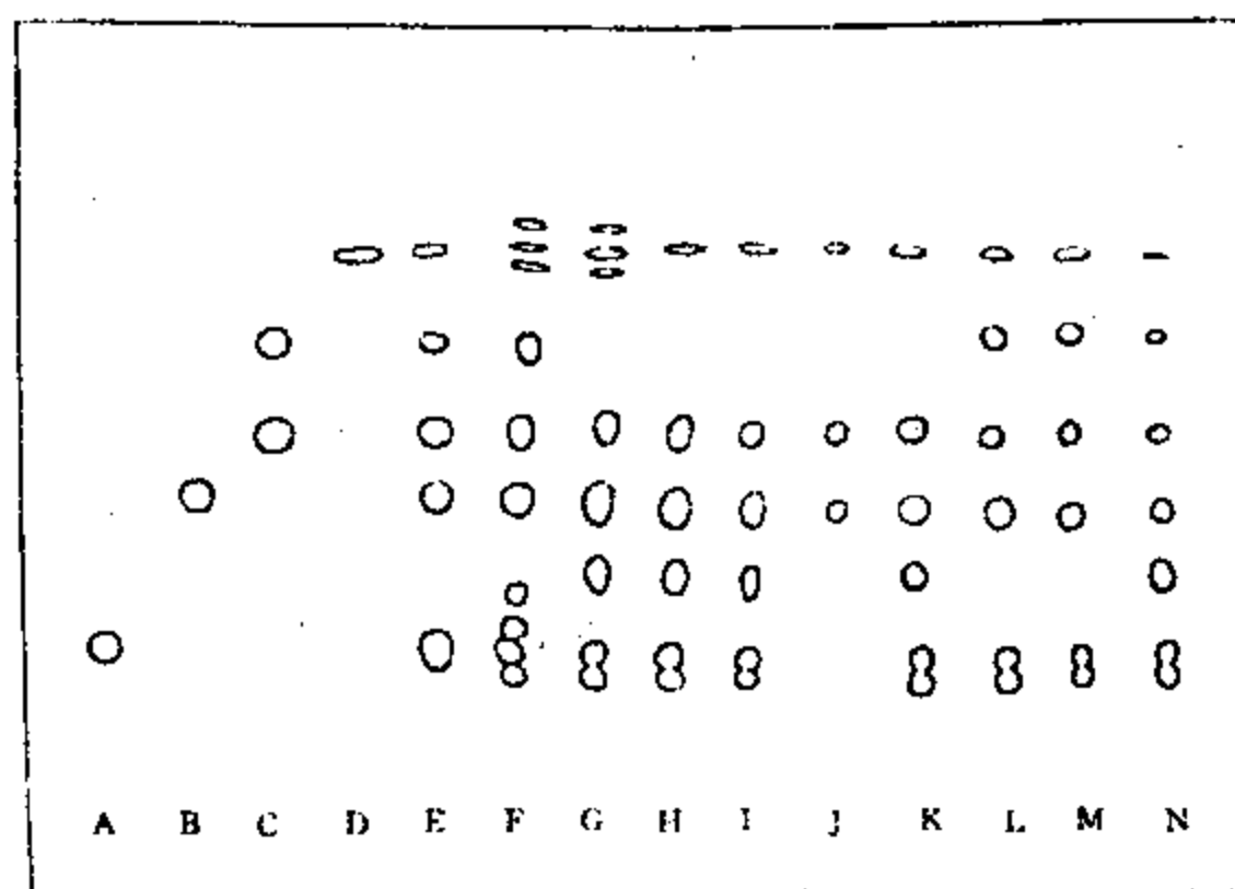
图 12-3-1 葛根异黄酮标准品与样品色谱图 展开剂 (I); UV254nm 紫外灯下观察 A. 大豆甙元-4'-7-二葡萄糖甙; B. 葛根素; C. 大豆甙; D. 大豆甙元; E. 异黄酮混合物; F. 生药 (四川峨边山); G. 生药 (江苏); H. 生药 (河北兴隆); I. 生药 (湖南长沙); J. 生药 (广东); K. 生药 (北京怀柔); L. 生药 (广西靖县); M. 生药 (广西桂林); N. 生药 (山东)
