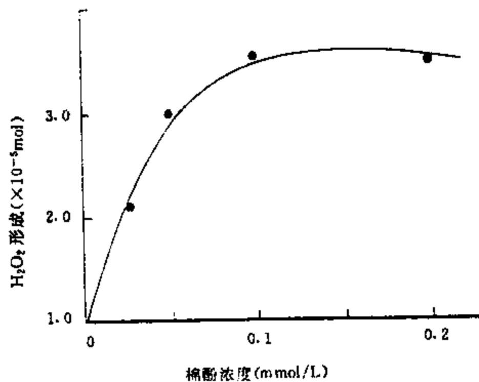
图 8-4-6 不同浓度醋酸棉酚引起 H 2 O 2 的形成
