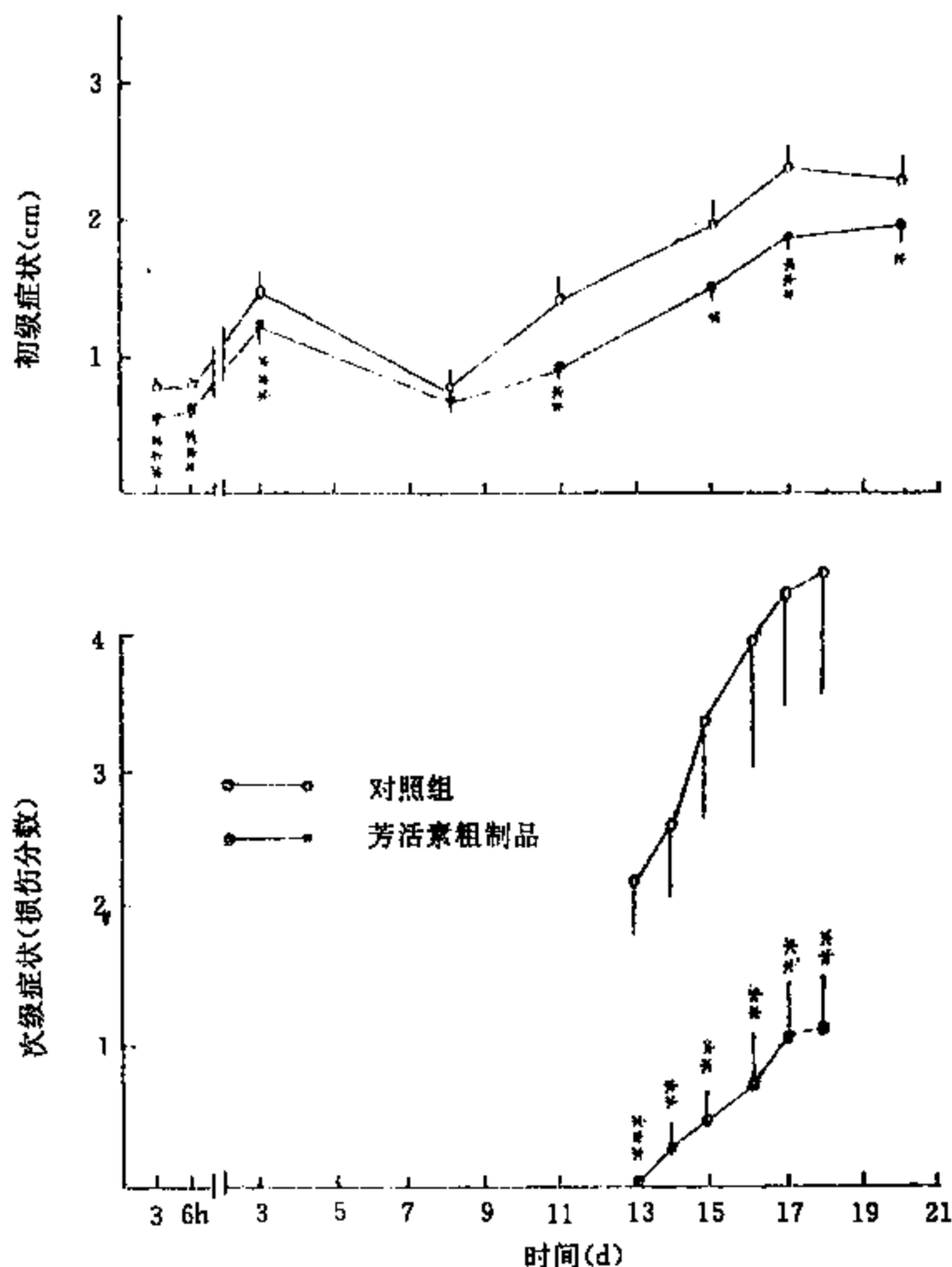
图 10-4-4 芳活素粗制品对大鼠佐剂型关节炎的作用 (* P < 0.05 , ** P < 0.01 , *** P < 0.001 )
