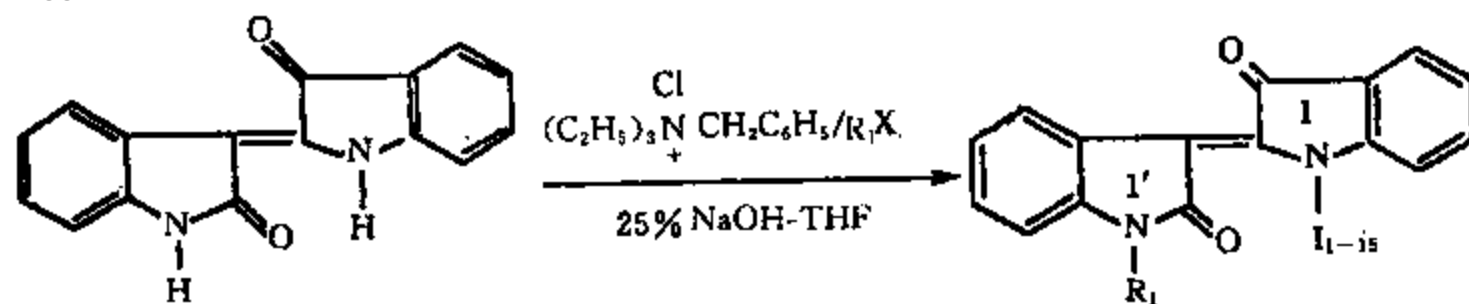
图 11-2-4 靛玉红衍生物 I_1 \sim I_{15} 的合成路线
