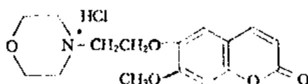
图 11 7-甲氧基-6-吗啉乙氧基香豆素 (盐酸盐 75018) 结构
