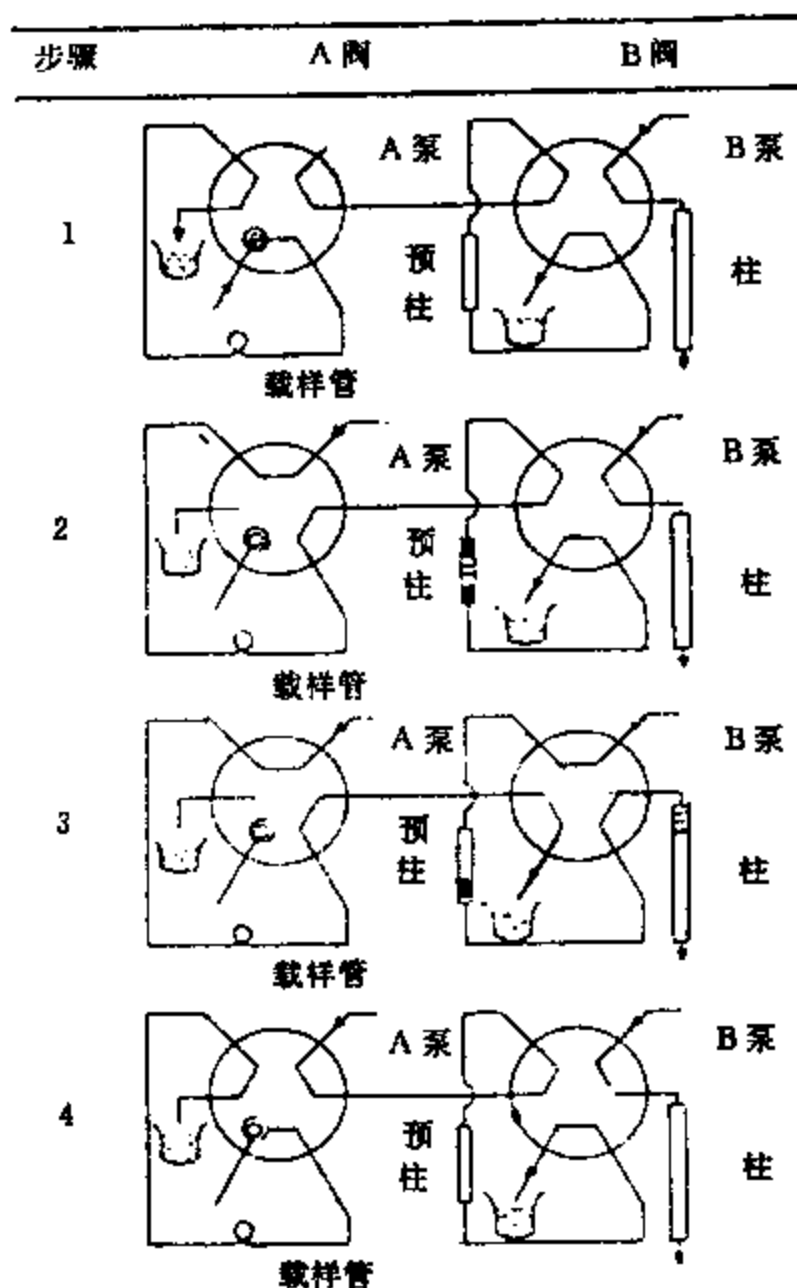
图 8-3-5 棉酚的柱切换分析程序
