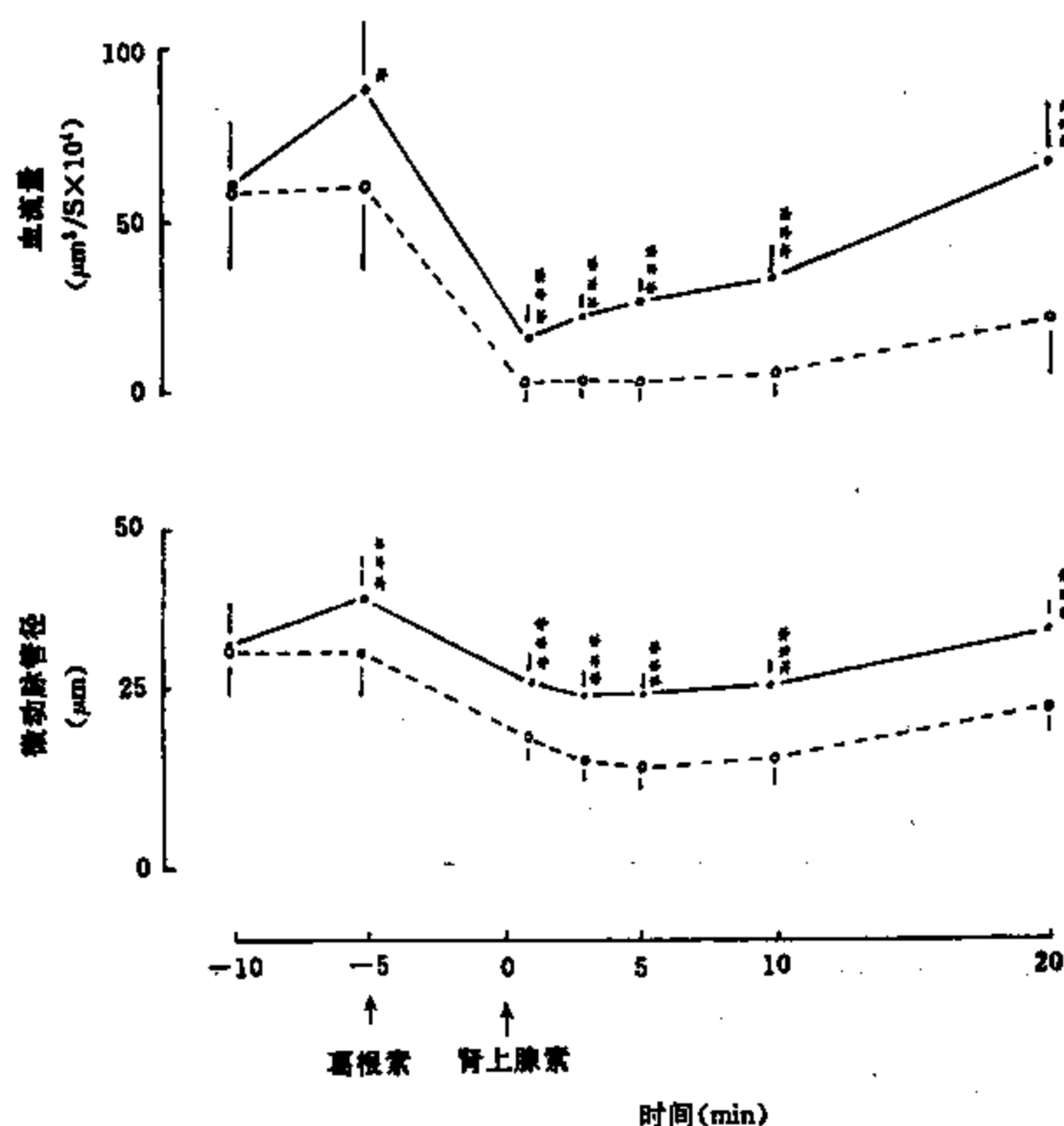
图 12-4-7 葛根素对肾上腺素引起小鼠肠系膜微循环障碍的影响
