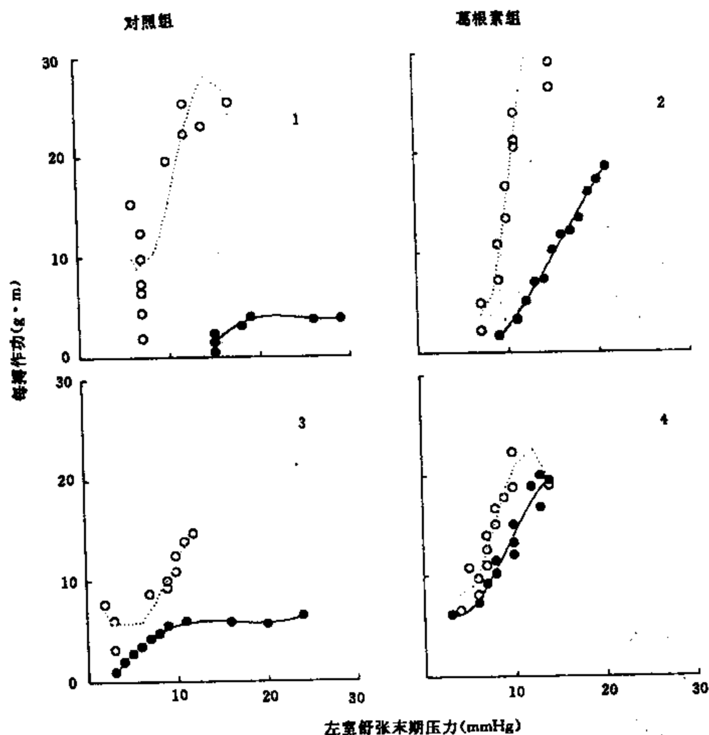
图 12-4-6 葛根素对体外循环狗心脏功能曲线的影响 对照组：停搏时用停搏液灌流心脏 葛根素组：停搏时用含有葛根素 2mg/kg·次的停搏液灌流心脏 .....停搏前的心脏功能曲线；——再灌流时的心脏功能曲线 图中 1, 2, 3, 4 代表动物号
