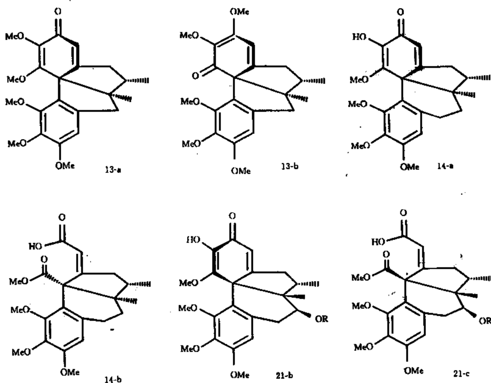
图 15 上-2-4 联苯环辛烯类木脂素碳键环化产物
