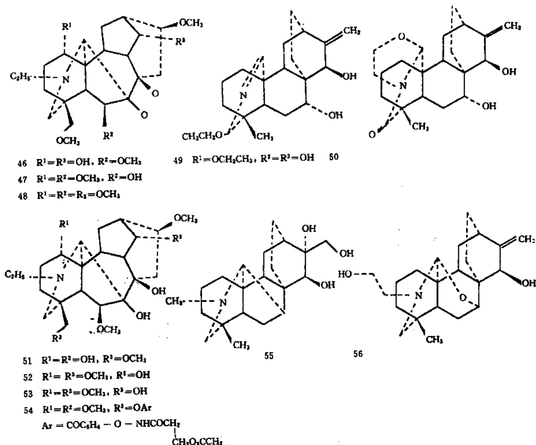
图1-2-15 囊翠碱甲(46)囊翠碱乙(47)囊翠碱丙(48)囊翠碱丁(49)囊翠碱戊(50)及化合物(51—56)的结构
