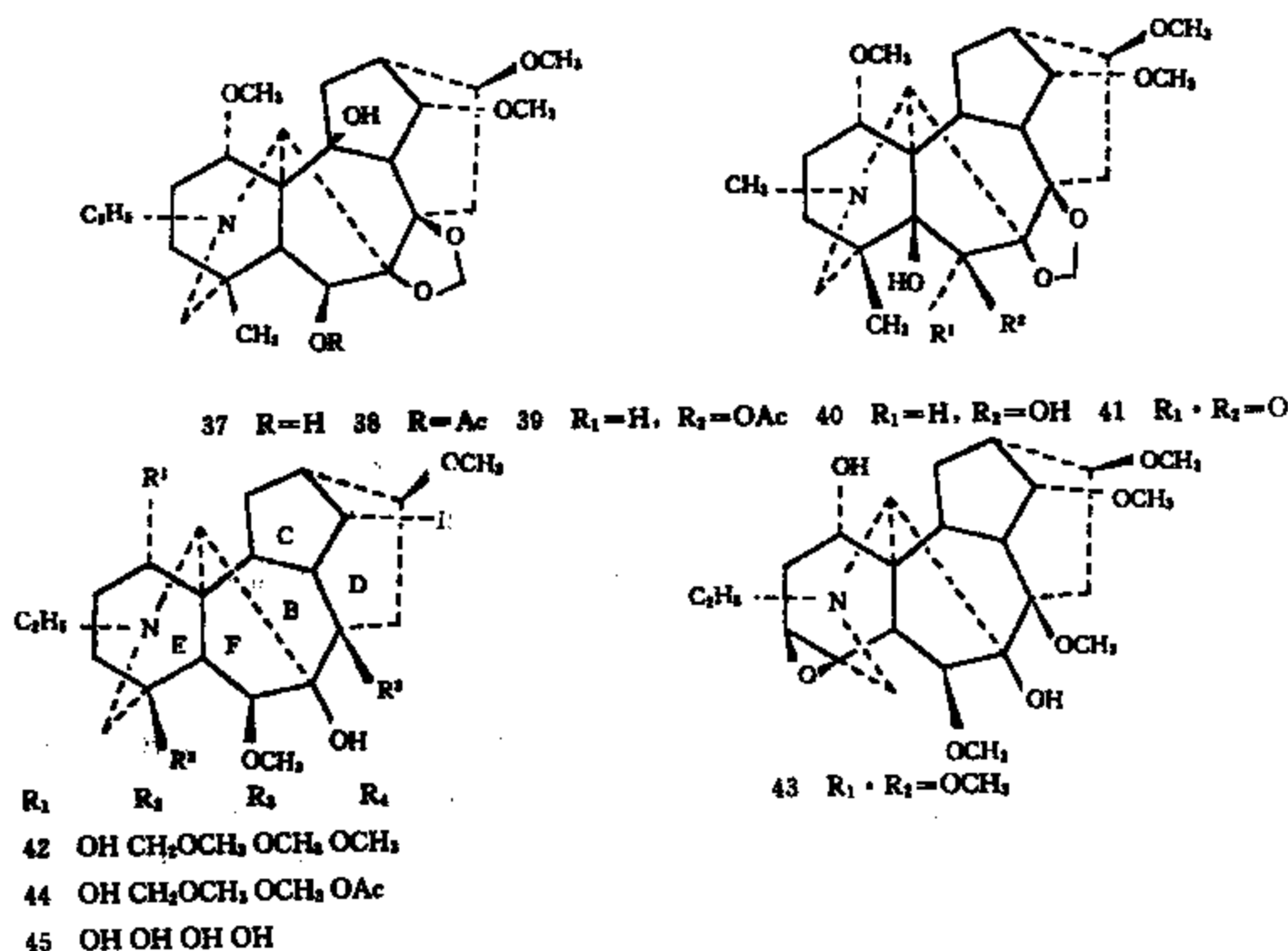
图 1-2-14 翠雀它明 (37) 翠雀它林 (38) 川翠碱甲 (39) 川翠碱乙 (40) 川翠碱丙 (41) 川翠碱丁 (42) 川翠碱戊 (43) 川翠碱己 (44) 川翠碱庚 (45) 的结构
