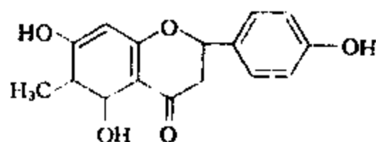
去甲杜鹌素
