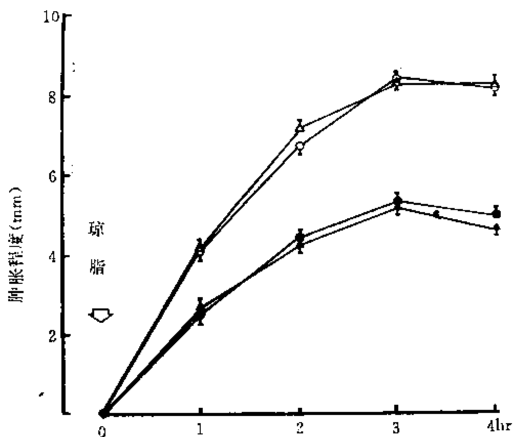
图 10-3-6 麝香对去垂体大鼠琼脂性关节肿的作用
