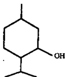
薄荷醇
