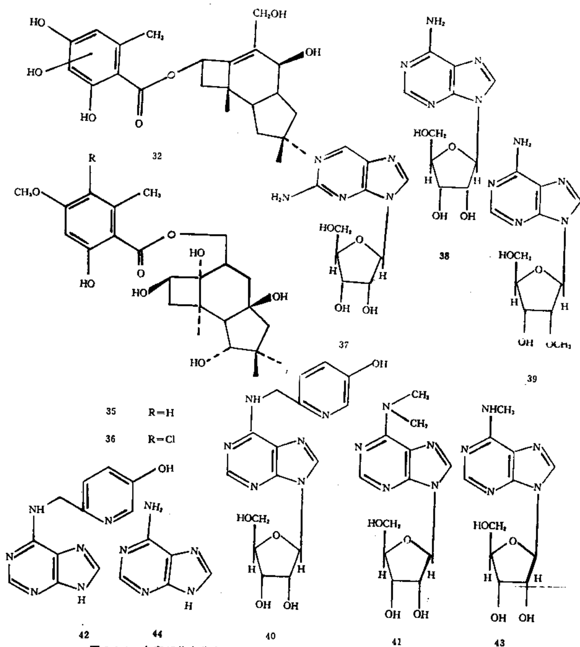
图 2-3-1 自蜜环菌中分离得到的原伊鲁烷倍半萜类和嘌呤类化合物的结构
