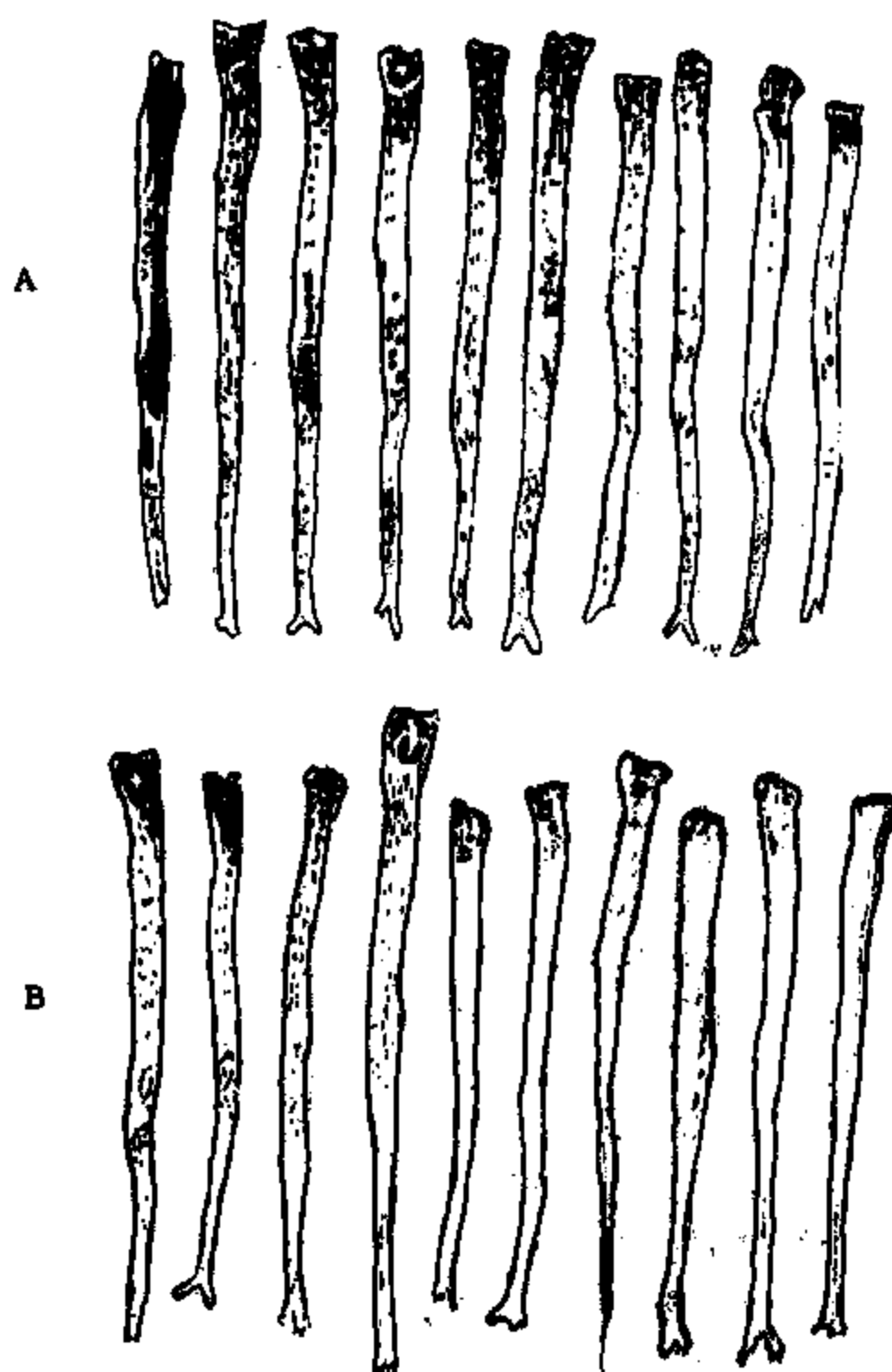
图 4-5-1 CsB 对饲高胆固醇兔主动脉壁粥样斑块形成的影响
