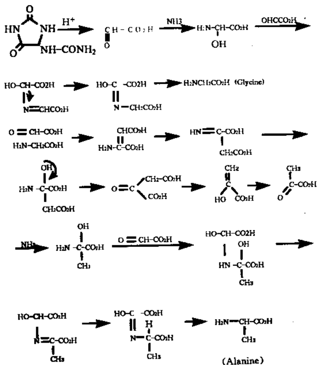
图 10-2-3 氨基酸形成的机制
