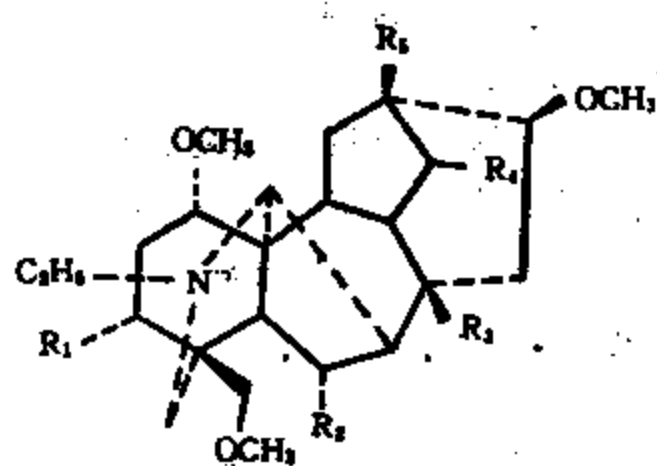
图 1-2-7 异叶乌头碱 (10) 苯甲酰异叶乌头碱 (11), 阿替辛 (12), 大麦芽碱 (13) 及唐乌碱 (14) 的结构
