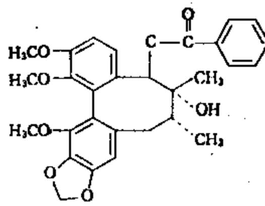
五味子酯甲
