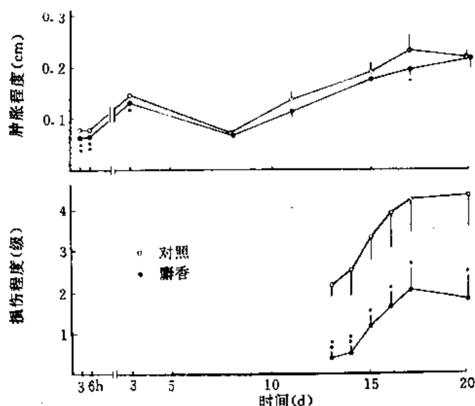
图 10-3-3 麝香对大鼠佐剂型关节炎的作用 (* P < 0.05 , ** P < 0.01 )
