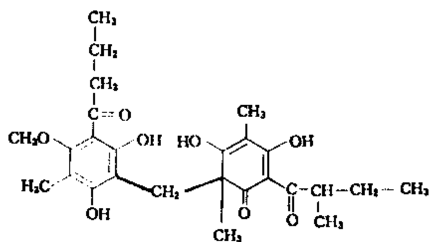
鹤草酚
