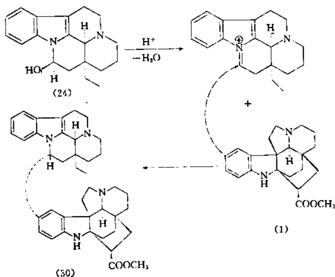
图 9-2-5 云南蕊木双碱的半合成
