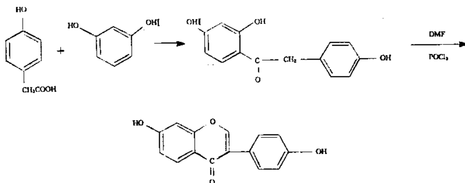
图 12-2-2 大豆甙元的合成路线
