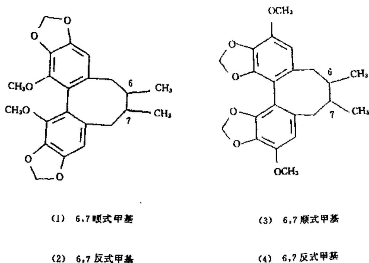
图 15 下-1-1 五味子丙素 (1) 及其同分异构体 (2, 3, 4) 的结构式
