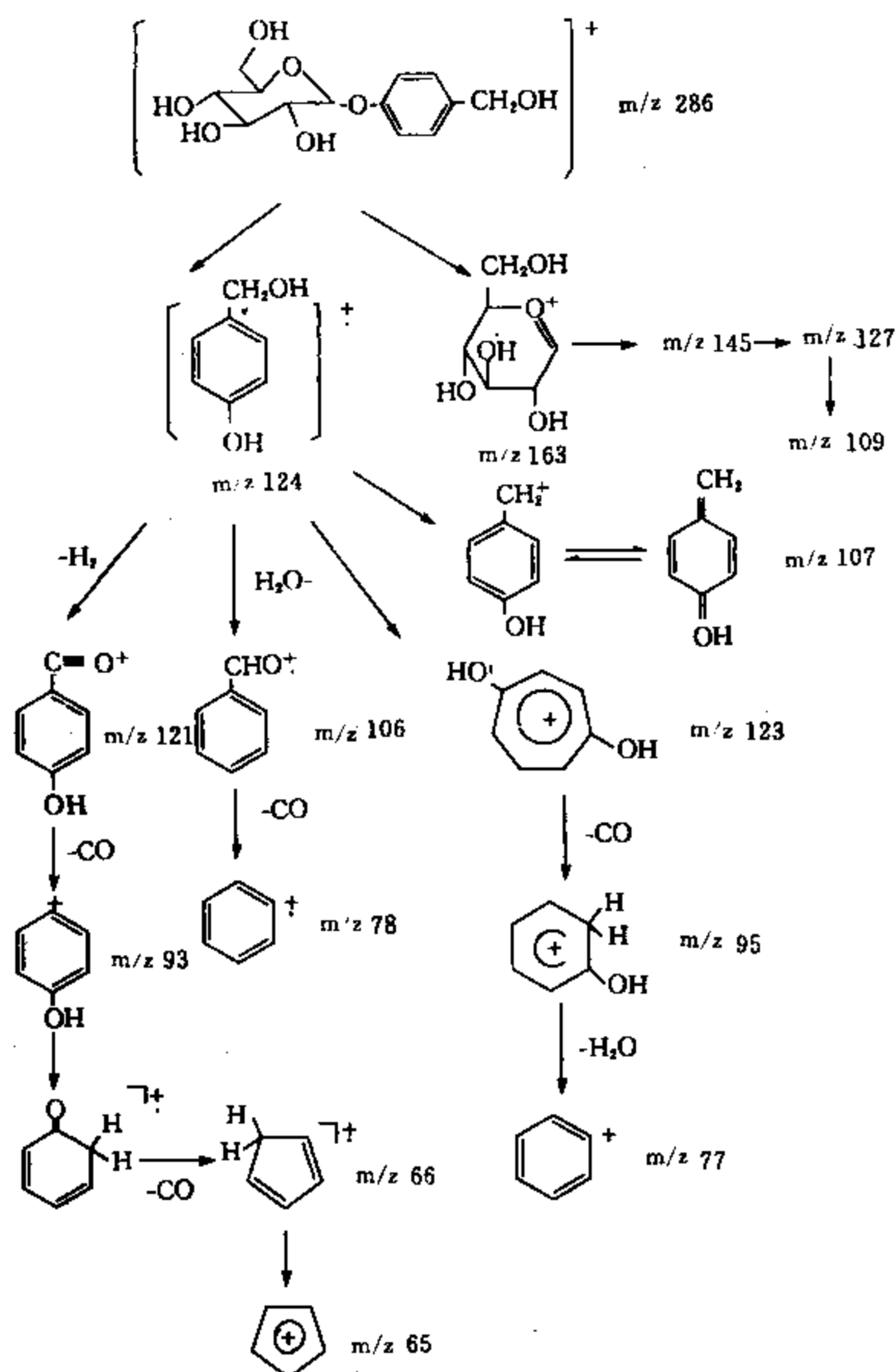
图 6-3-2 天麻甙质谱裂解图
