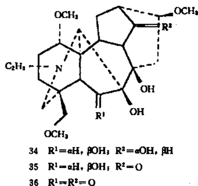
图 1-2-13 鞘乌甲素 (34) 鞘乌乙素 (35) 和鞘乌丙素 (36) 的结构
