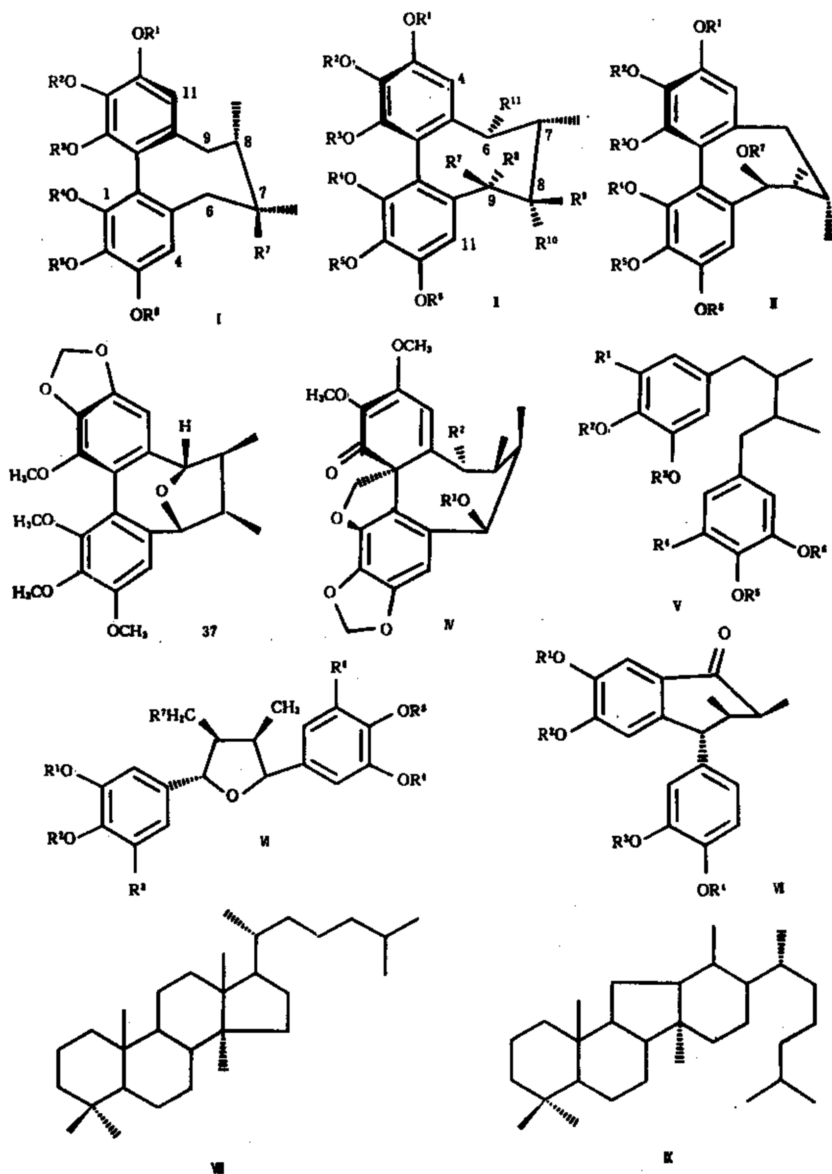
图 15 上-2-1 木脂素和三萜类的结构骨架
