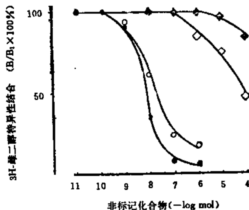
图 8-4-4 己烯雌酚 (•—•), 雌三醇 (0—0), 醋酸棉酚 (□—□) 和 15 甲基 \text{PGF}_{2\alpha} 甲酯 (■—■) 与 ^3\text{H} -雌二醇竞争性结合大鼠子宫雌激素受体
