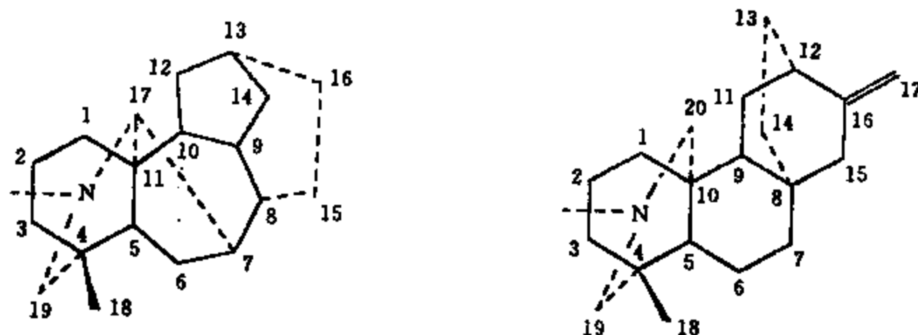
图 1-2-1 C_{19} -乌头碱型骨架 C_{20} -阿替辛型骨架
