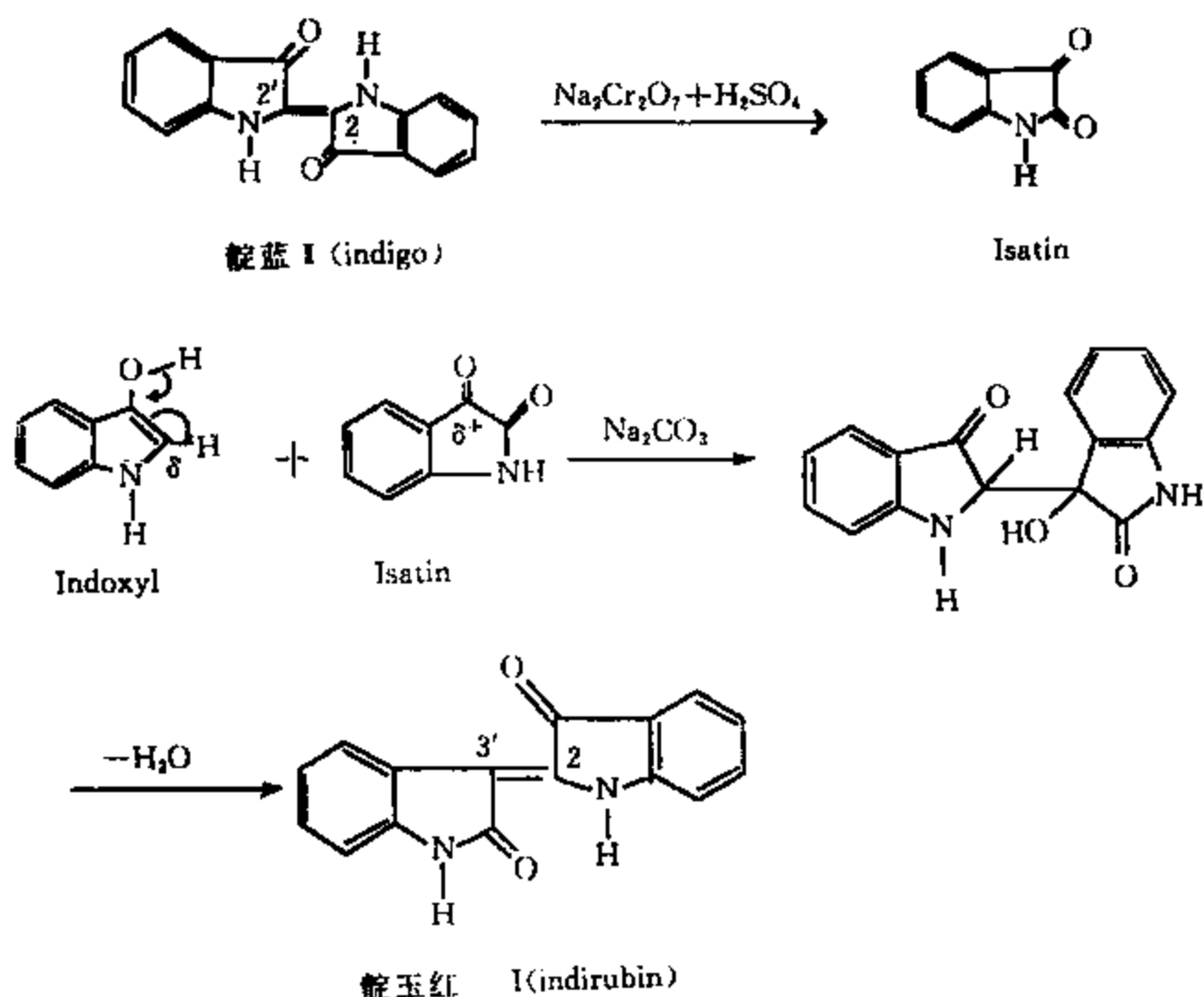
图 11-2-3 靛玉红的全合成路线
