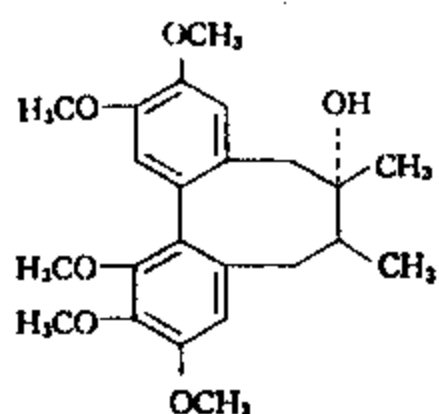
五味子乙素
