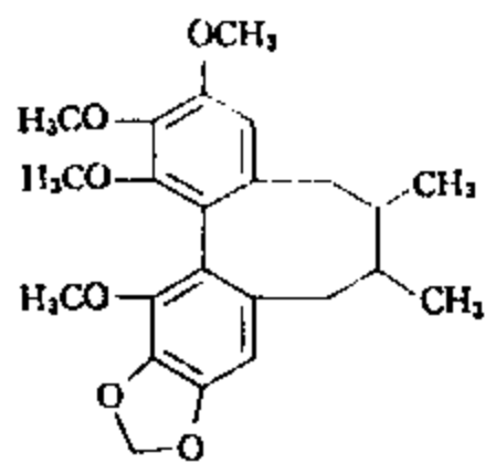
五味子乙素
