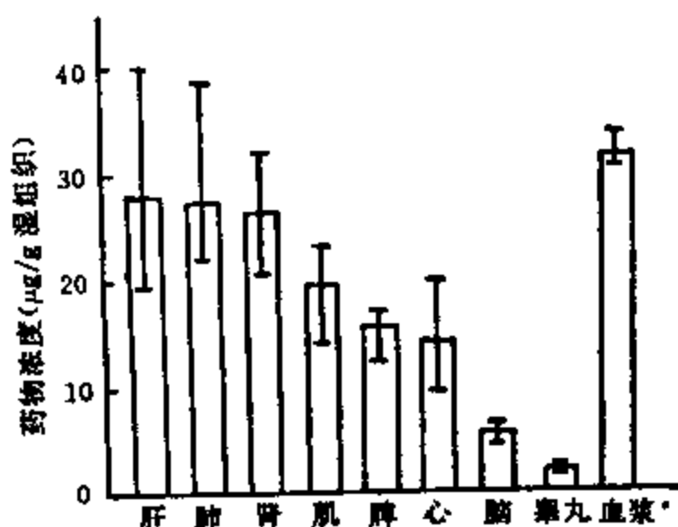
图 12-6-6 大豆甙元在组织的分布
