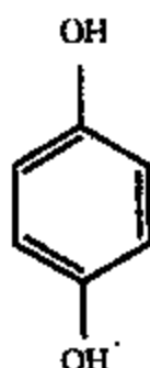
氢醌
