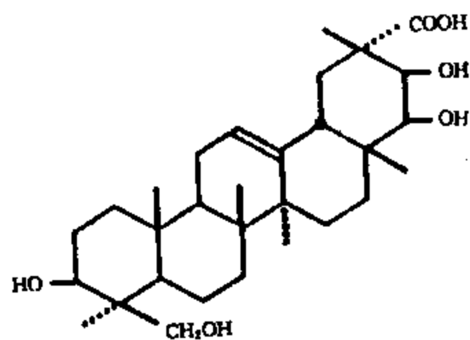
28 葛根甙元 B
