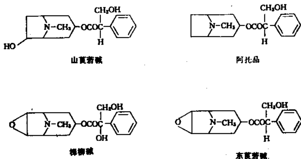
图1 山莨菪碱和樟柳碱结构
