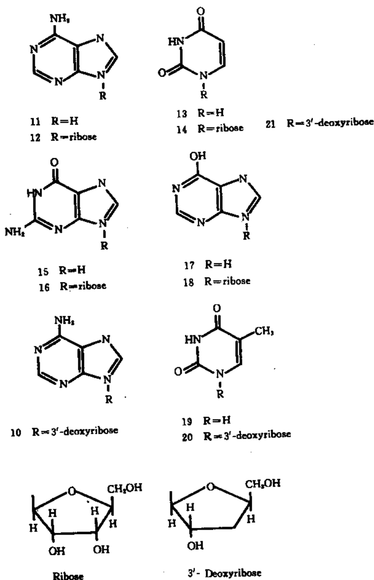
图 4-3-2 冬虫夏草和人工虫草核苷类化合物（10—21）结构
