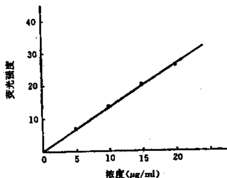
图 12-6-11 葛根素在大鼠血浆中的标准曲线 \lambda_{ex} : 355nm; \lambda_{em} : 473nm
