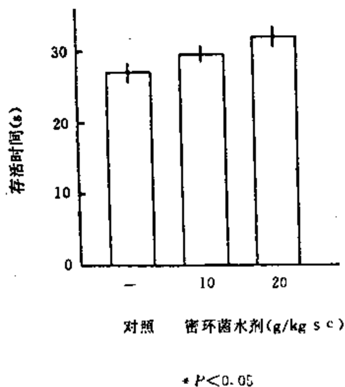
图 2-4-4 蜜环菌水剂对氰化钾 (KCN) 缺氧的影响
