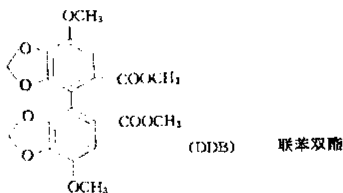
图 8 联苯双酯结构
