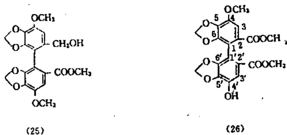
图 15 下-2-4 联苯双酯衍生物 (25) 和 (26) 结构图
