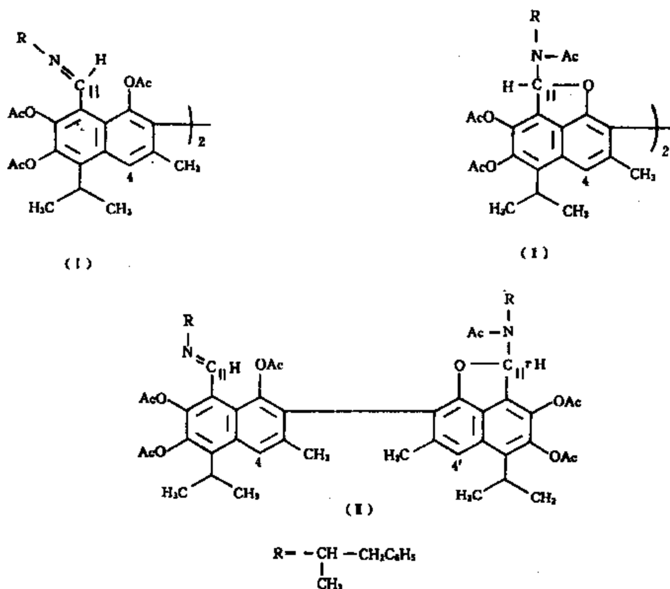
图 8-2-7 胺缩棉酚六乙酸酯的同分异构体
