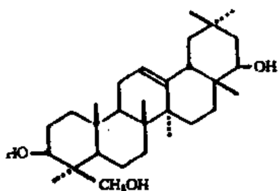
24 大豆甙元 B
