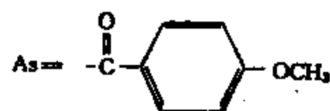
图 1-2-8 展花乌头宁 (15) 它拉乌头胺 (16) 滇乌碱 (17) 粗茎乌碱甲 (18) 和黄花乌碱丙 (19) 的结构
