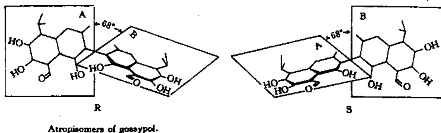
图 8-2-5 棉酚手性分子
