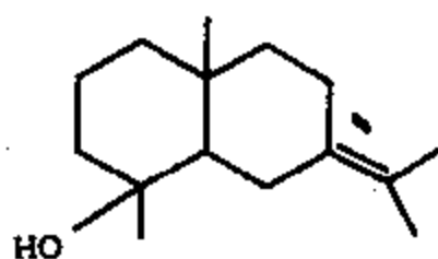
杜松脑
