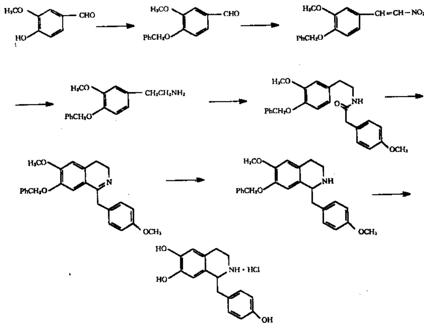
图 1-3-1 附子一号合成路线
