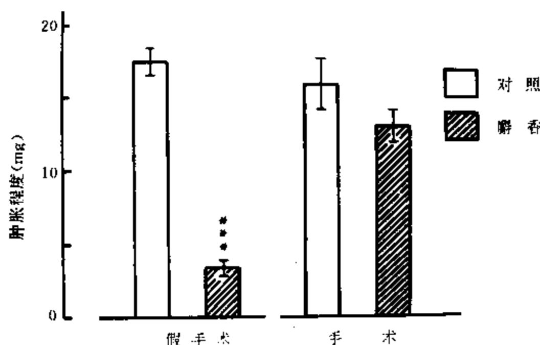
图 10-3-5 肾上腺切除对麝香抗炎作用的影响 (巴豆油引起小鼠耳部炎症, *** P < 0.001 )
