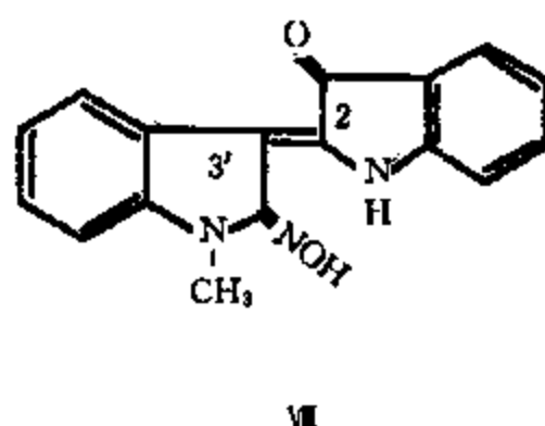
图 11-2-9 N -甲基靛玉红衍生物的结构
