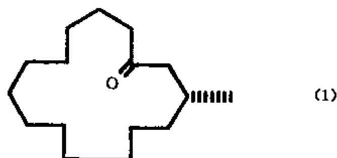
图 10-2-1 麝香酮的结构
