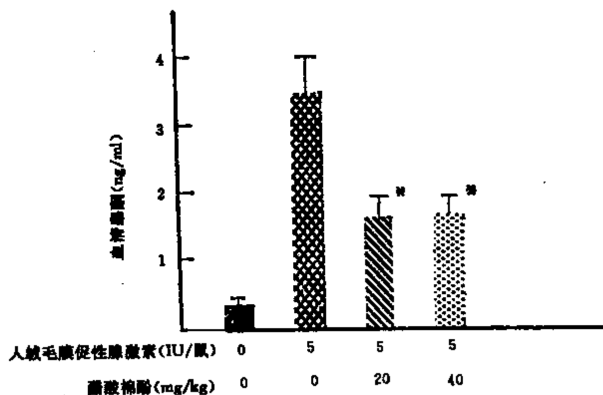
图 8-4-3 棉酚对幼大鼠血清睾酮水平的影响
