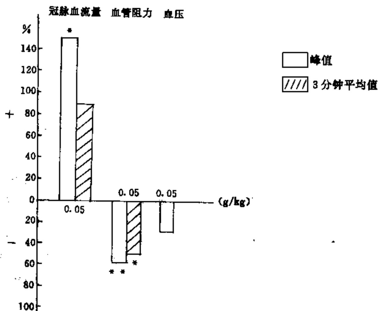
图 2-4-5 动脉注射蜜环菌水剂 (g/kg) 对麻醉犬冠状循环血流动力的作用
