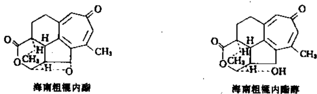
图4 海南粗榧内酯及海南粗榧内酯醇结构
