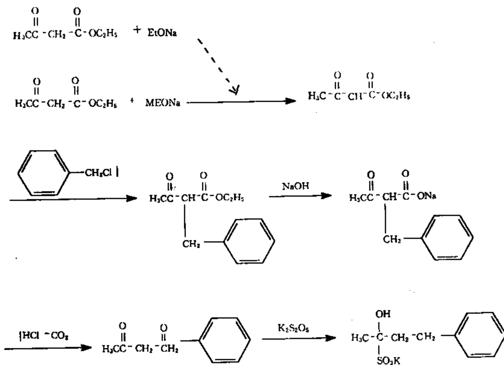
图 14-3-6 改良的止咳酮合成路线
