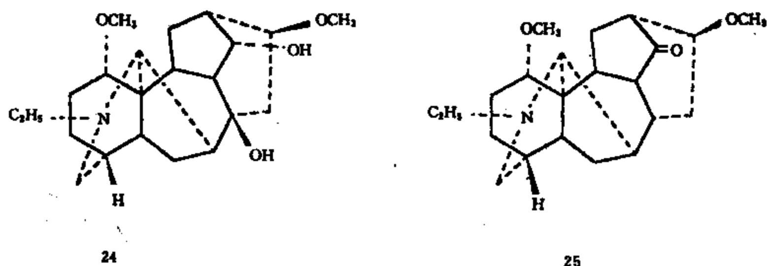
图 1-2-10 阿康诺辛 (24) 脱氧脱氢阿康诺辛 (25) 的结构
