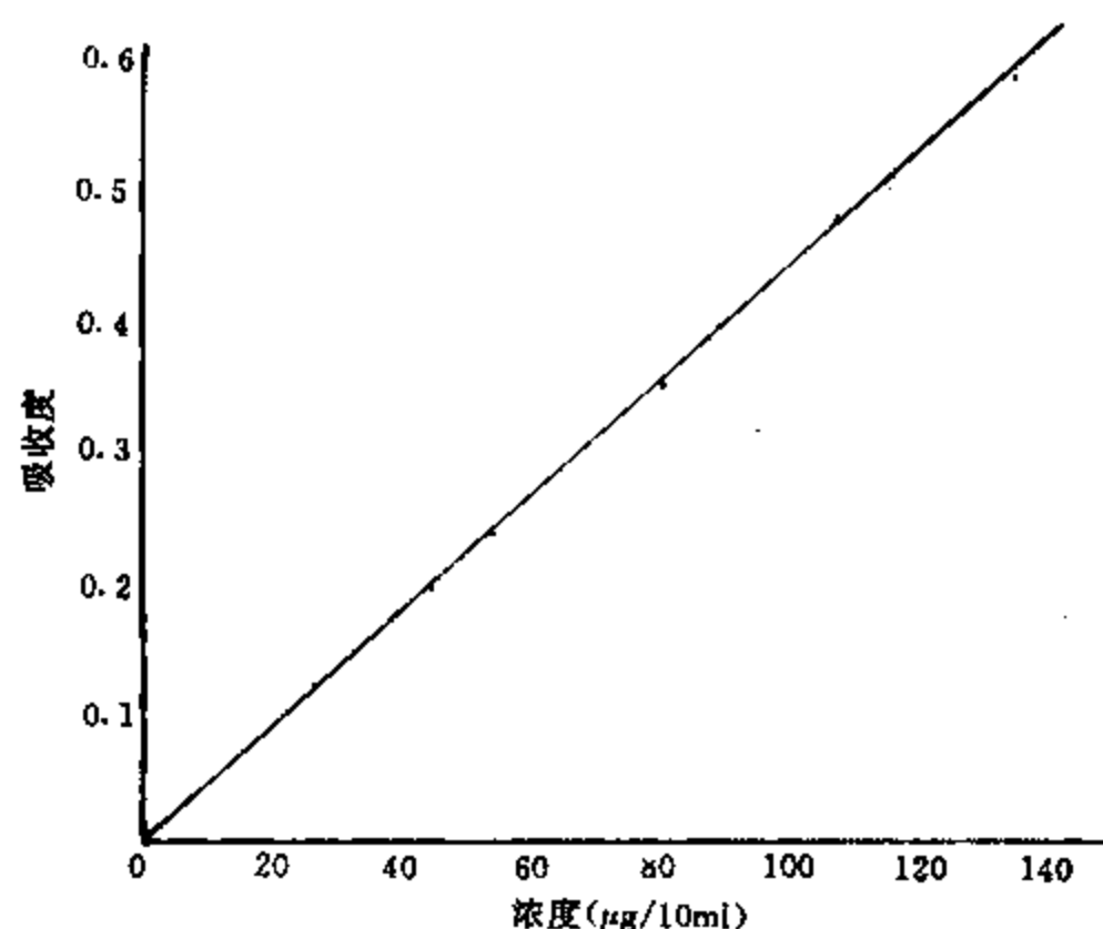
图 11-3-1 靛玉红浓度与吸收度关系曲线
