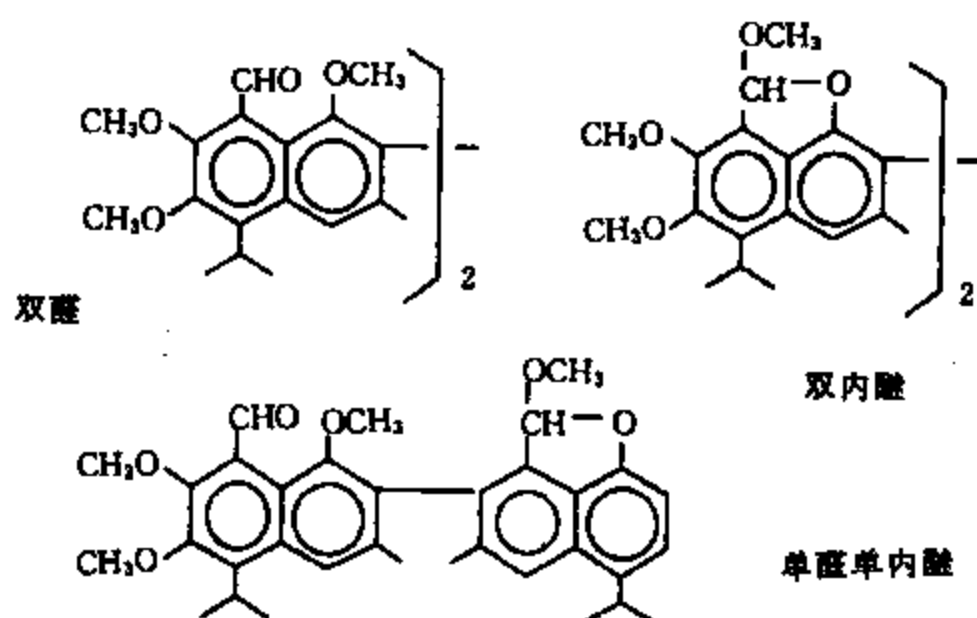
图 8-2-2 棉酚六甲醚的三种同分异构体
