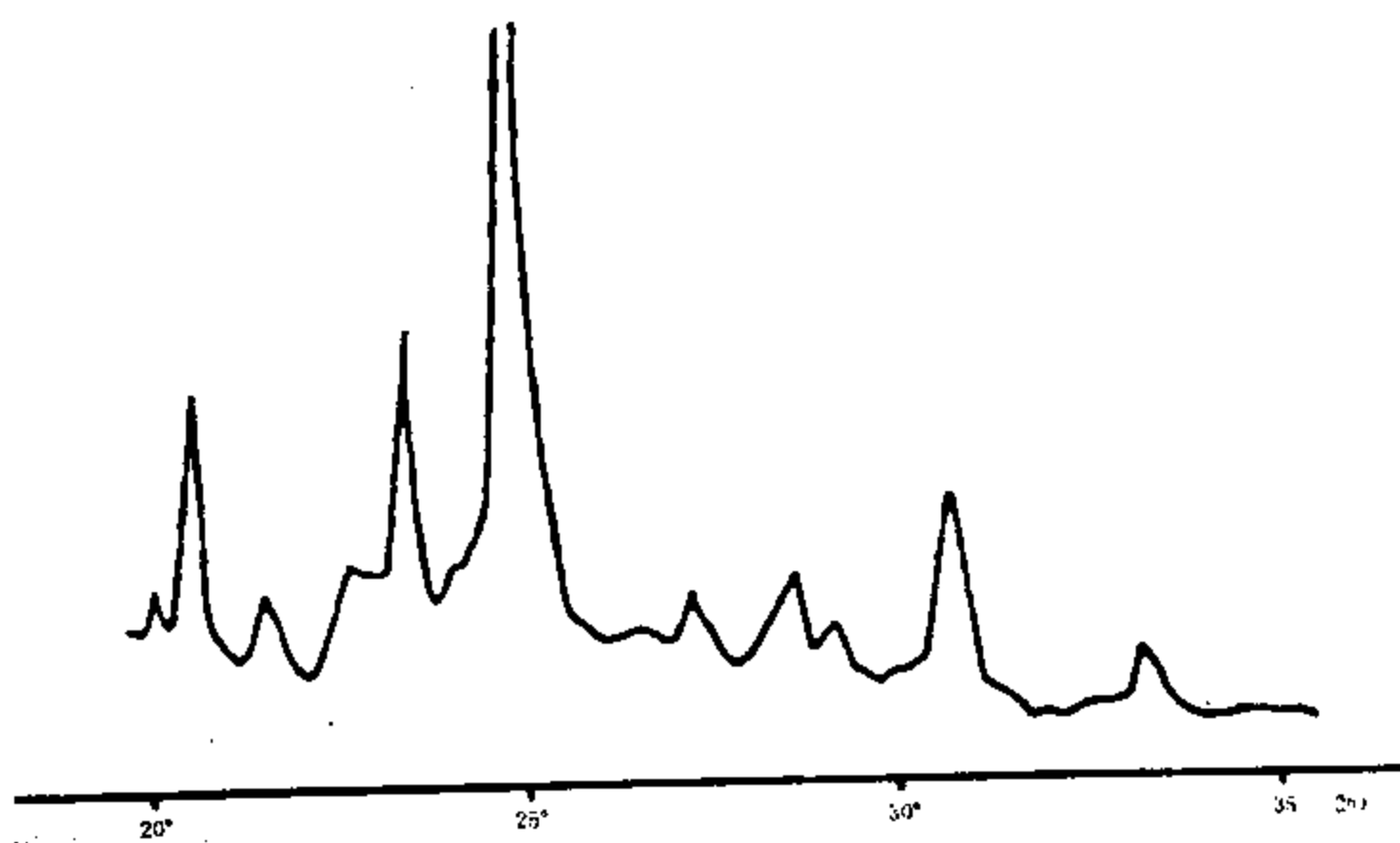
图 15 下-4-1 联苯双酯 X-射线衍射图
