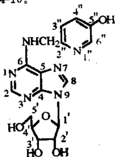
图 2-4-10 HPMA 的化学结构
