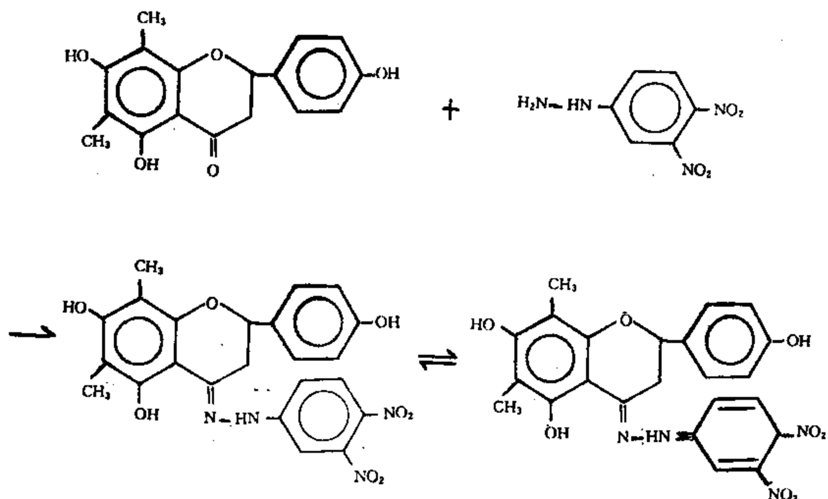
图 14-4-3 杜鹃素与 2,4-二硝基苯肼反应式
