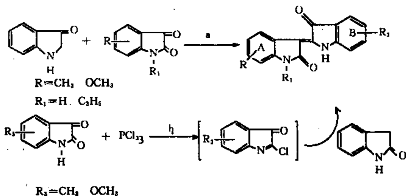
图 11-2-7 赭玉红苯环取代衍生物 (I 20~24 ) 的合成路线
