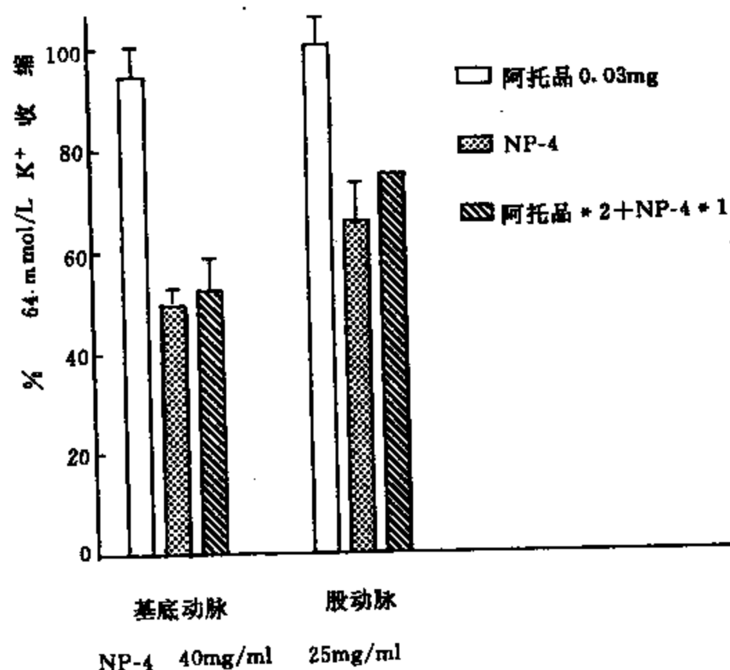
图 2-4-7 阿托品对 NP-4 对抗高钾收缩血管作用的影响
