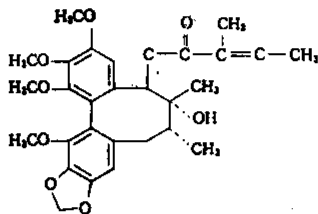
五味子酯乙
