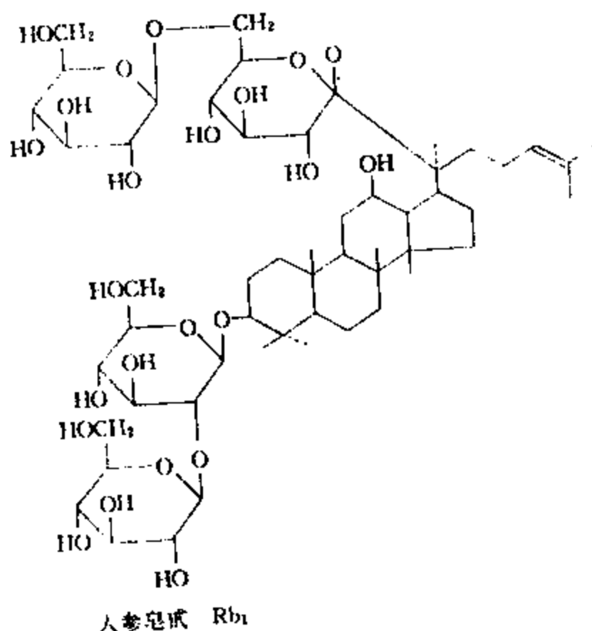
图 2 几种促智药结构
