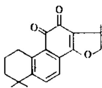
隐丹参酮
