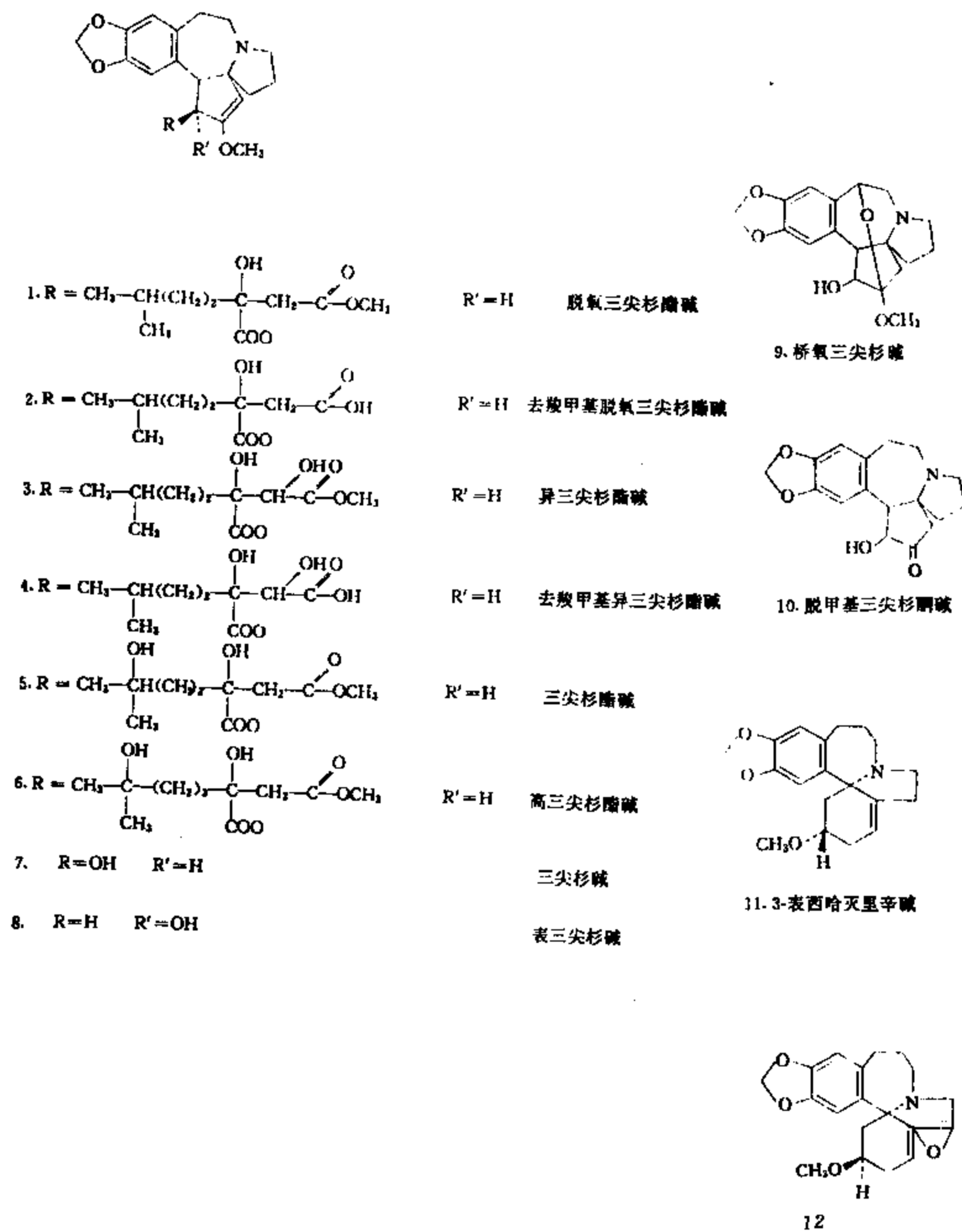
图3 三尖杉酯类生物碱结构
