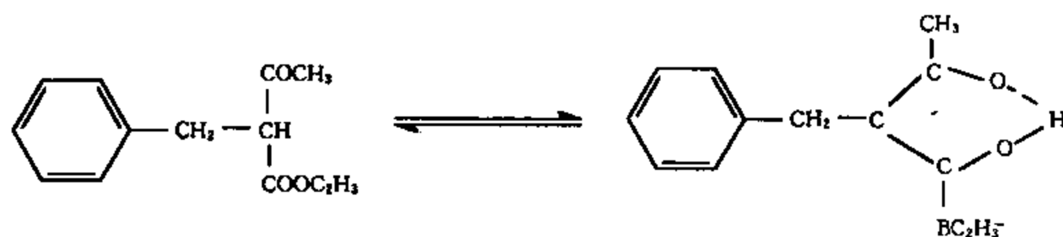
图 14-3-4 止咳酮合成路线
