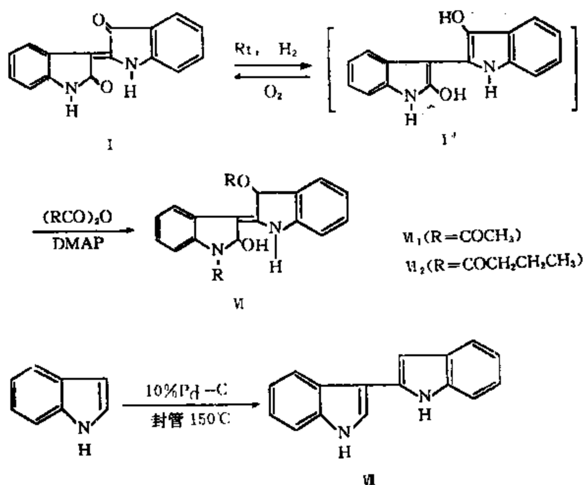
图 11-2-8 靛玉红分子中 2, 3' 位以单键相连的衍生物, 类似物的合成方法
