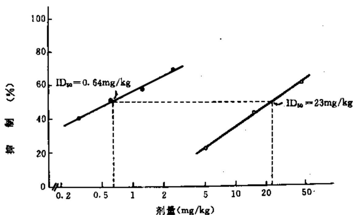
图 10-3-4 麝香-1 及氢化可的松对小鼠巴豆油耳炎的作用 ● 麝香-1, ○ 氢化可的松
