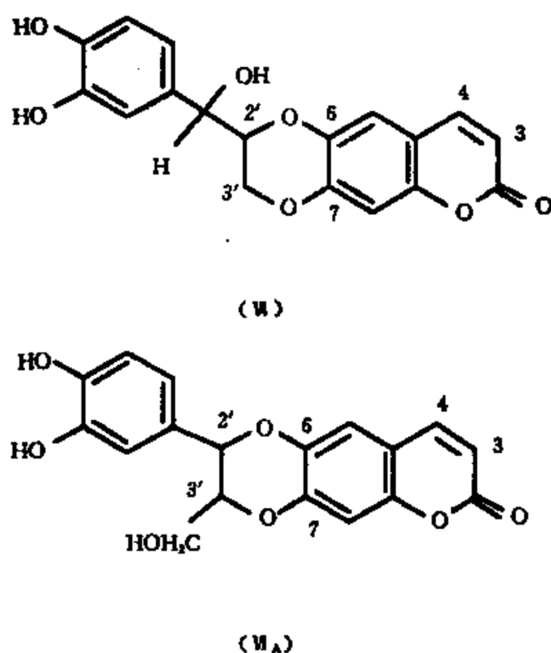
图 5-2-2 猫眼草素的结构
