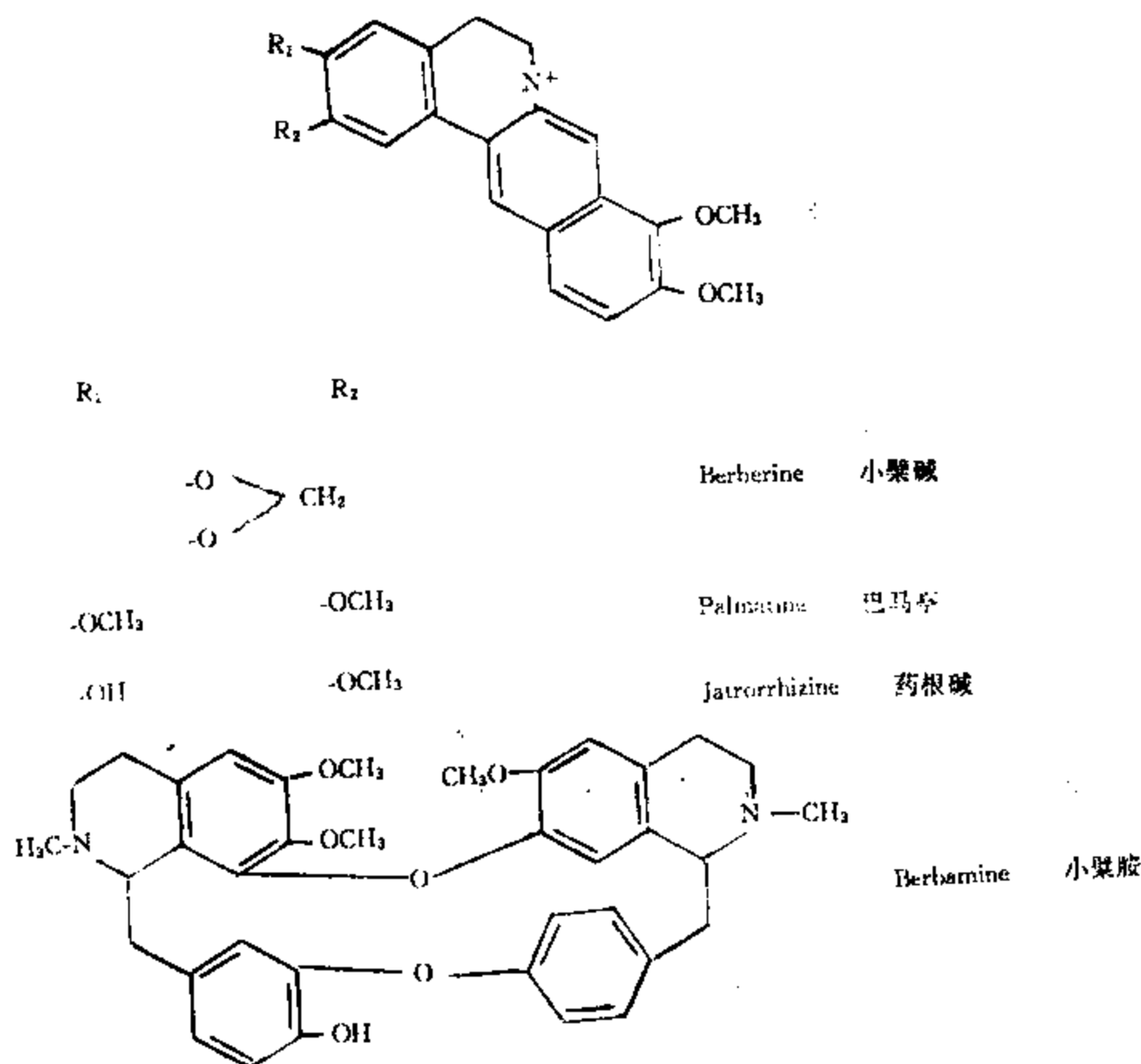
图 3-2-1 4 种生物碱的结构
