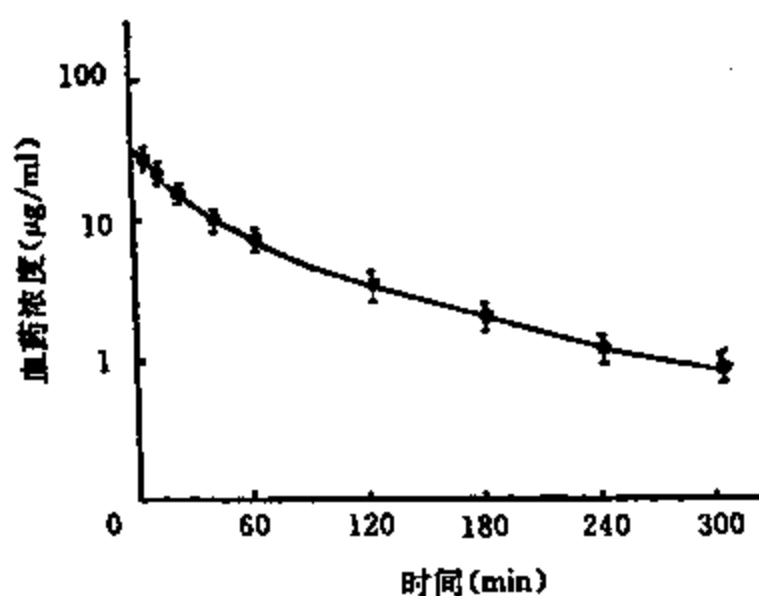
图 12-6-16 正常志愿者 iv 葛根素 5mg 后药-肘曲线
