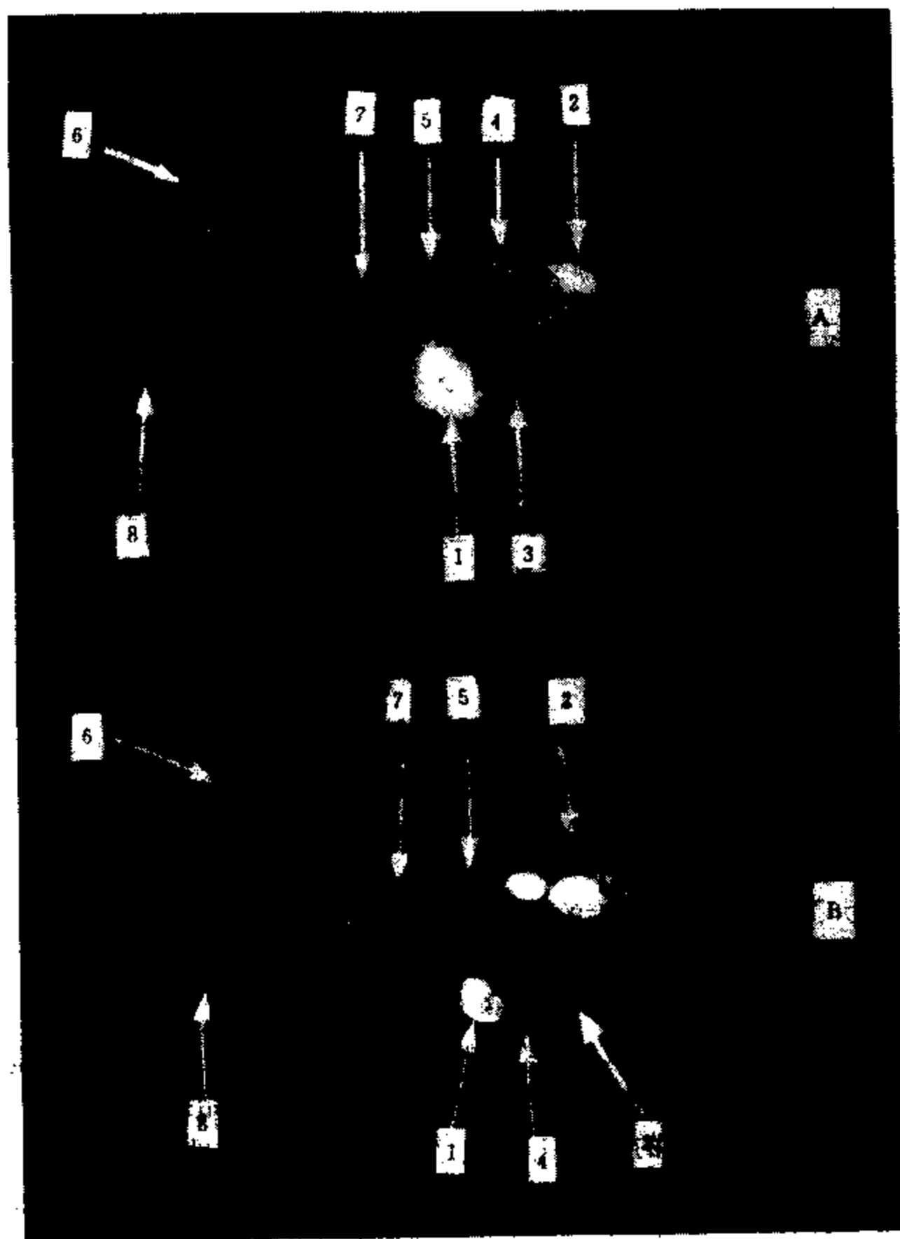
图 11-4-2 Lewis 肺癌小鼠口服 ^3\text{H} -甲异靛后的整体放射自显影
