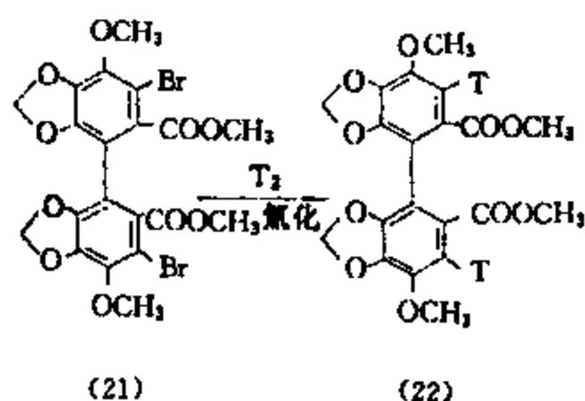
图 15 下-2-2 3 H-联苯双酯合成反应式
