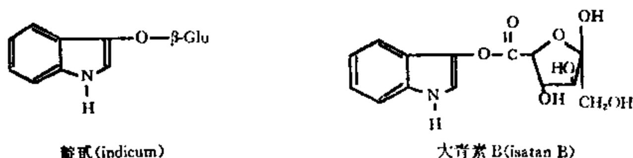
图 11-2-1 靛甙、大青素 B 的结构
