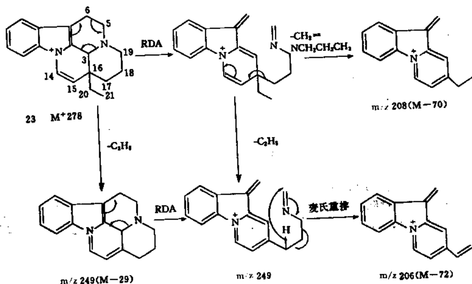
图 9-2-3 云南基木生物碱 (23) 质谱裂解
