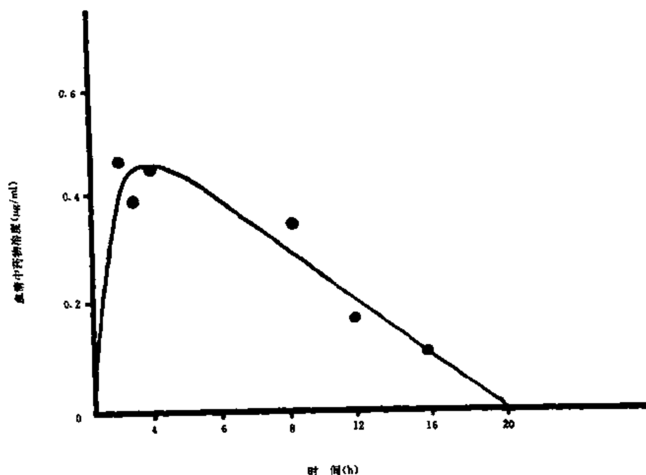
图 15 下-4-9 小鼠口服联苯双酯滴丸 50mg/kg 后的血清药溶度—时间曲线 (n=3)
