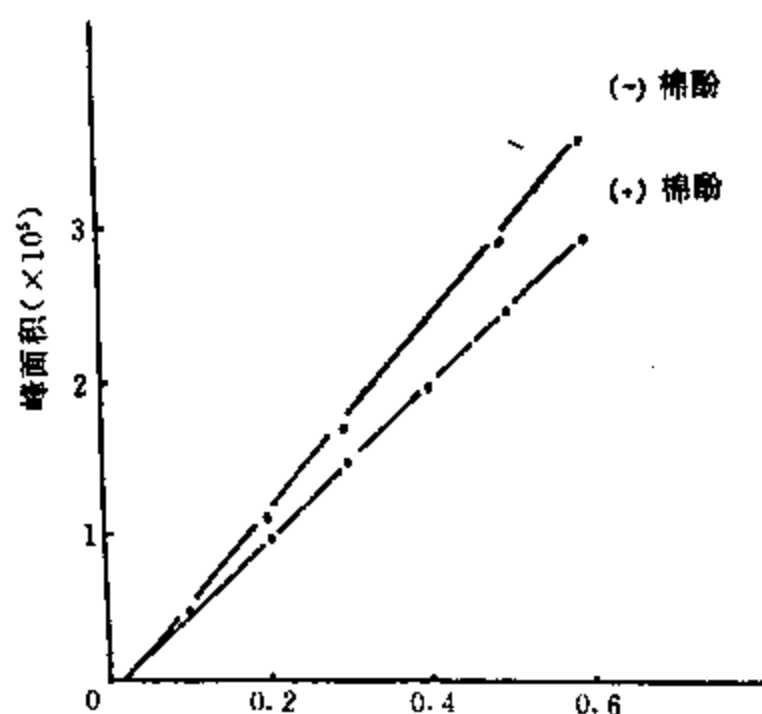
图 8-3-4 (+)、(-) 棉酚的标准曲线
