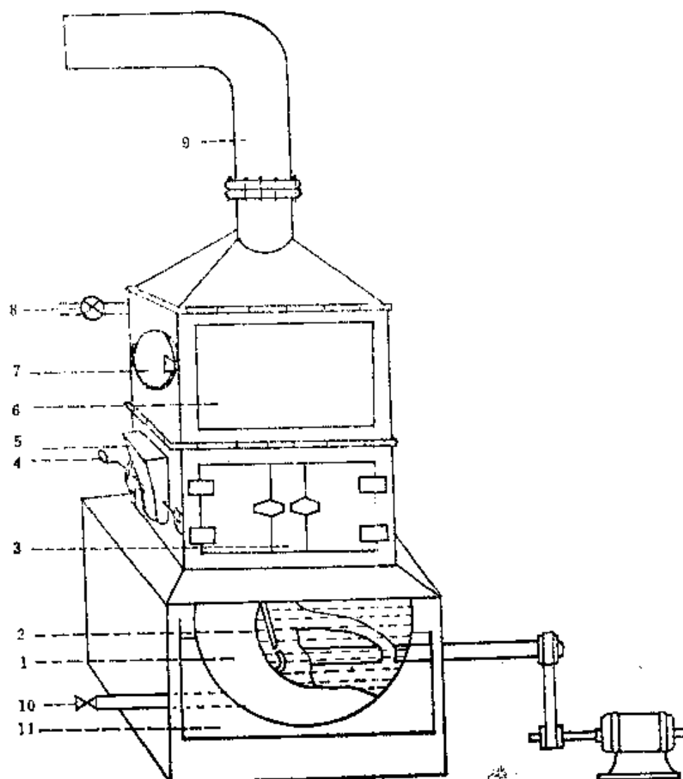
图12 膏药下丹锅简图
