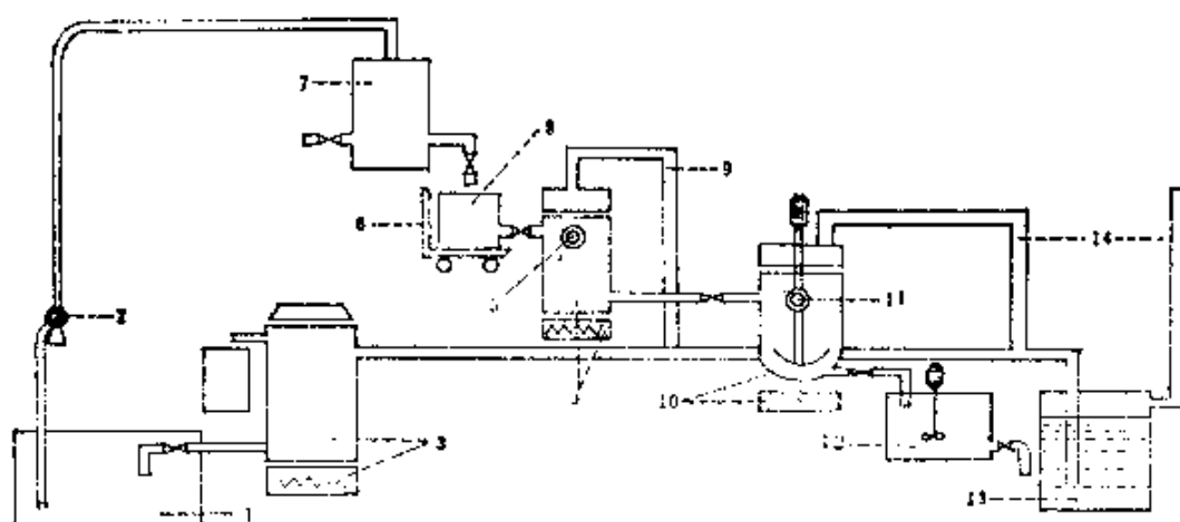
图13 大量生产黑膏药生产流程
