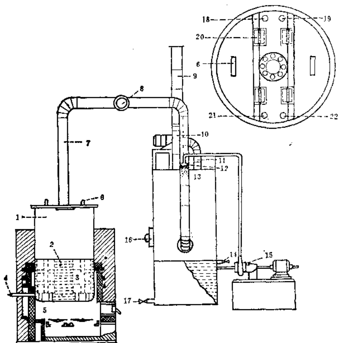
图11 膏药提取与炼油器简图
