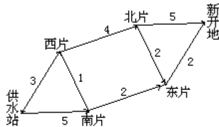
供水系统管路图
